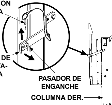
DESENGANCHAR LA PLATAFORMA DE LA COLUMNA IZQUIERDA FIG. 14-2
