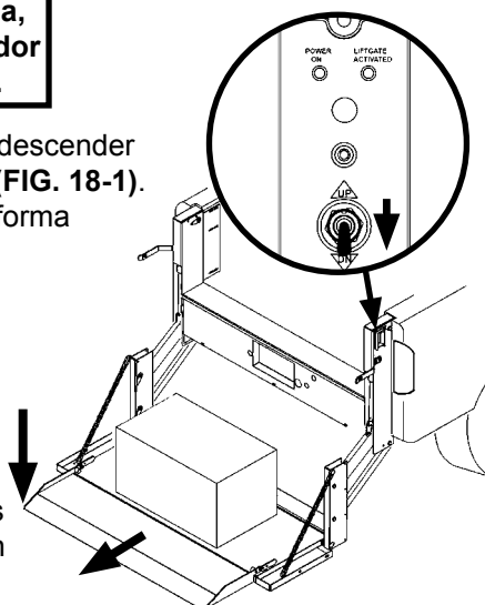
DESCARGAR PLATAFORMA AL NIVEL DEL SUELO FIG. 18-2
