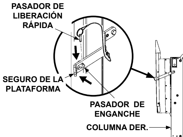
ENGANCHAR PLATAFORMA A LA COLUMNA DERECHA FIG. 20-1
