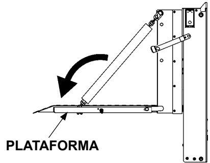
DESPLEGAR LA PLATAFORMA (VISTA LATERAL DERECHA)
