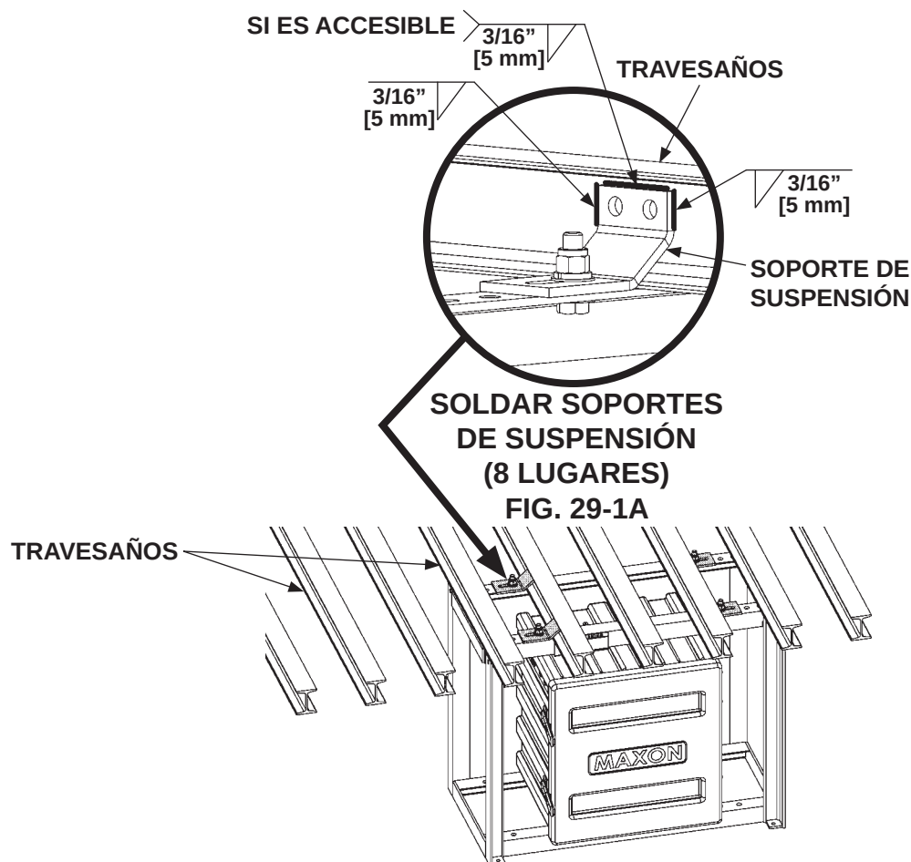
SOLDAR SOPORTES DE SUSPENSIÓN DEL MARCO A LOS TRAVESAÑOS DEL VEHÍCULO FIG. 29-1
