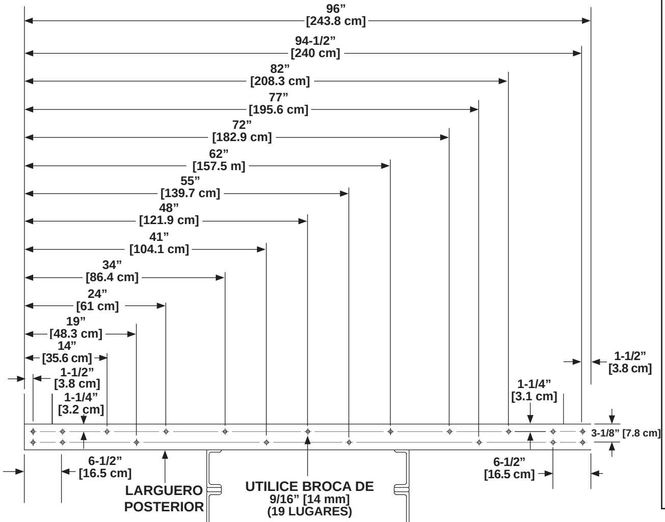
LARGUERO POSTERIOR - UBICACIÓN DE LOS ORIFICIOS EN VEHÍCULO DE 96" [243.8 cm] DE ANCHO
