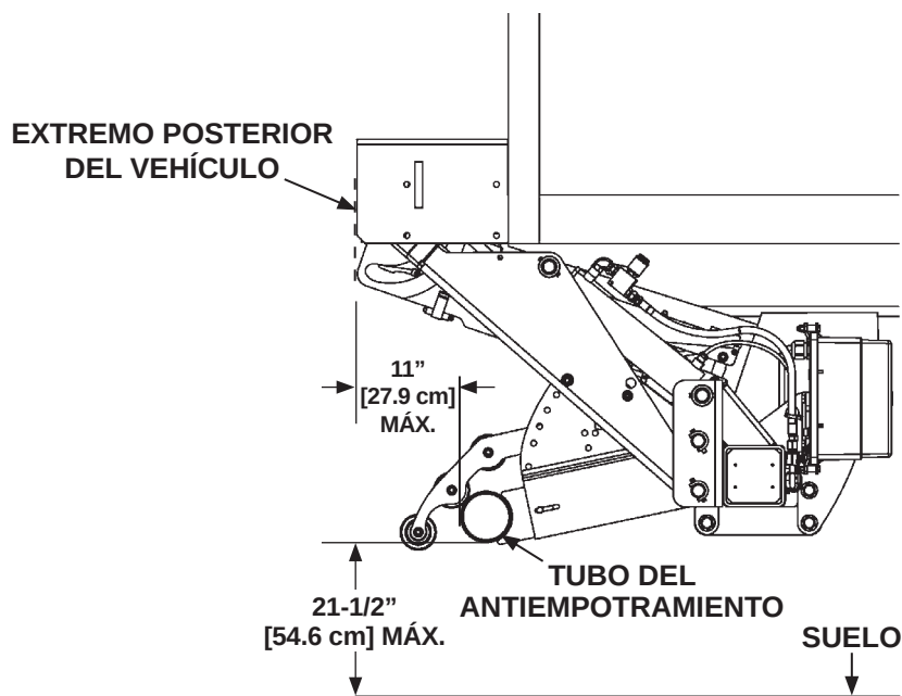
ELEVADOR GPTLR-44 Ó GPTLR-55, EQUIPADO CON DISPOSITIVO DE ANTIEMPOTRAMIENTO ESTÁNDAR, MOSTRANDO LOS ESPACIOS MÁXIMOS PERMITIDOS FIG. 65-1
