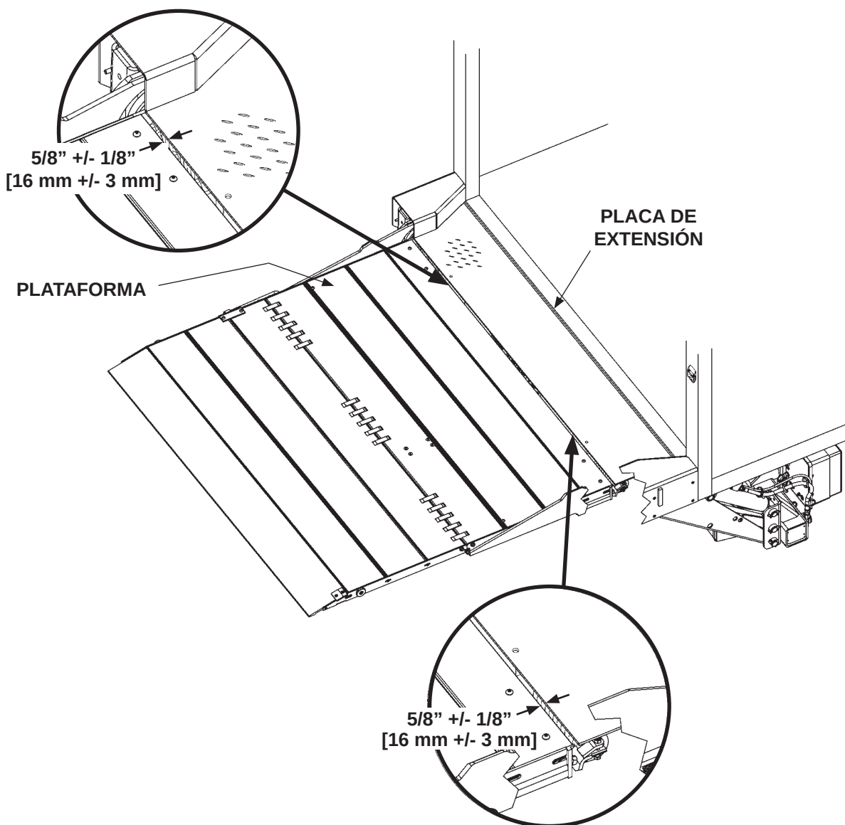
VERIFICAR EL ESPACIO ENTRE LA PLATAFORMA Y LA PLACA DE EXTENSIÓN FIG. 48-1
