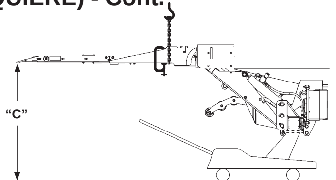
MEDIDAS DE ESPACIO PARA EL ELEVADOR FIG. 56-1
