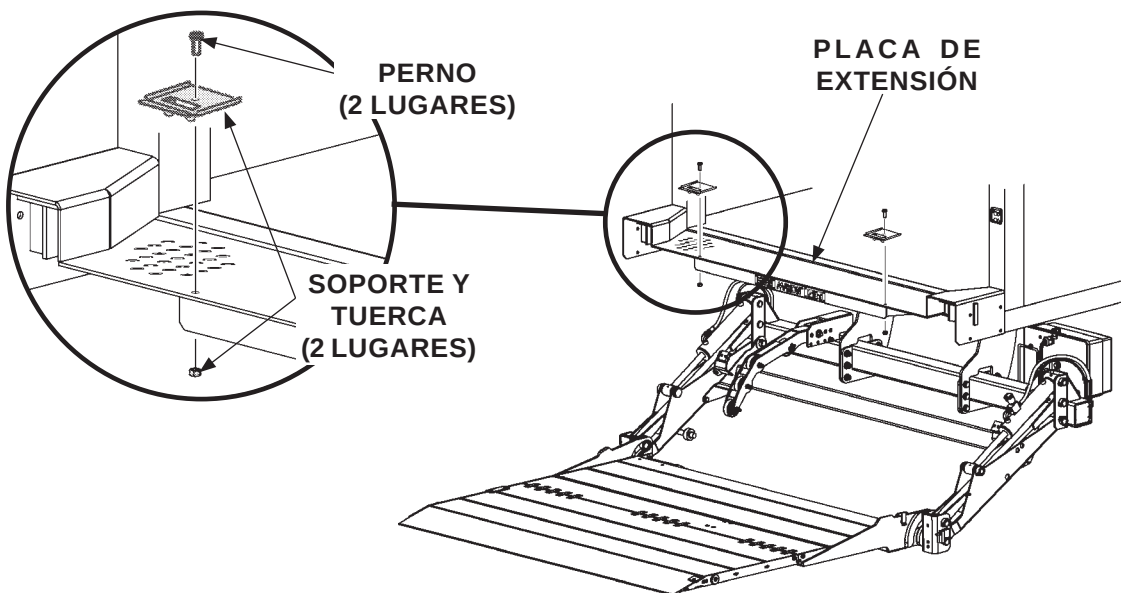
RETIRAR LOS SOPORTES DE SEGURIDAD FIG. 46-1
