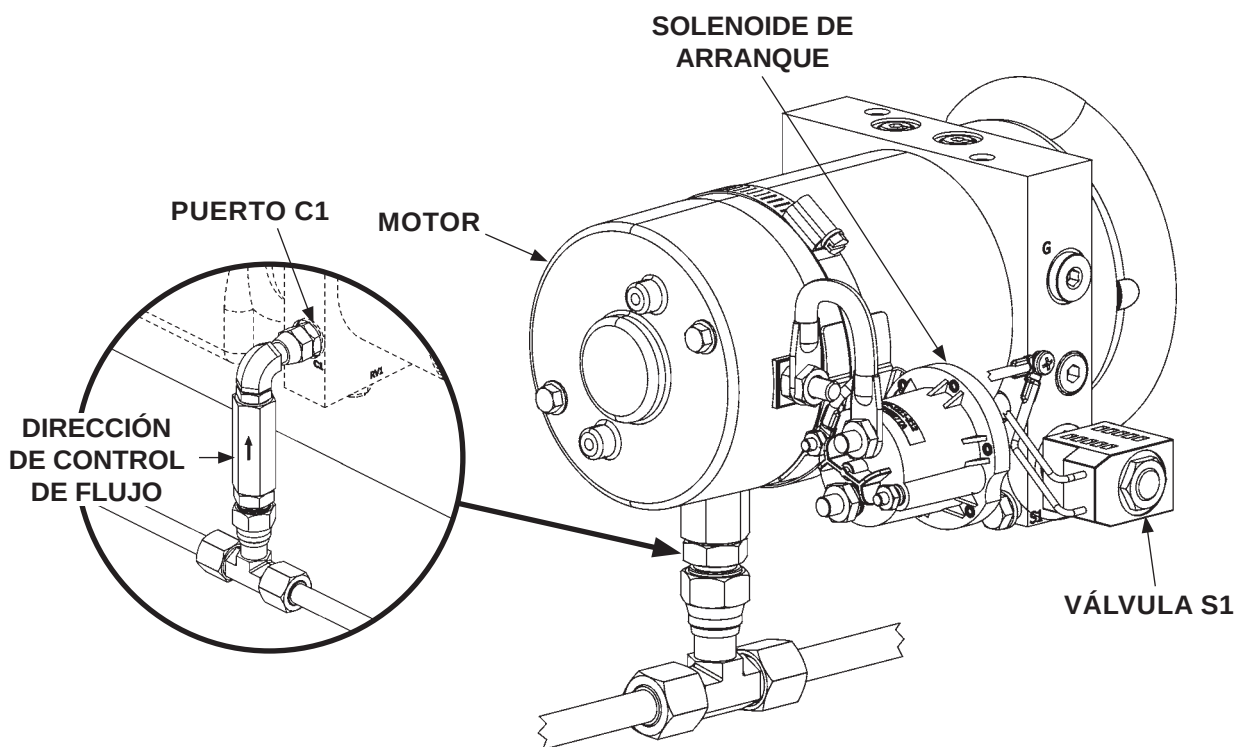
UNIDAD DE POTENCIA CON DESCENSO POR GRAVEDAD FIG. 84-1
