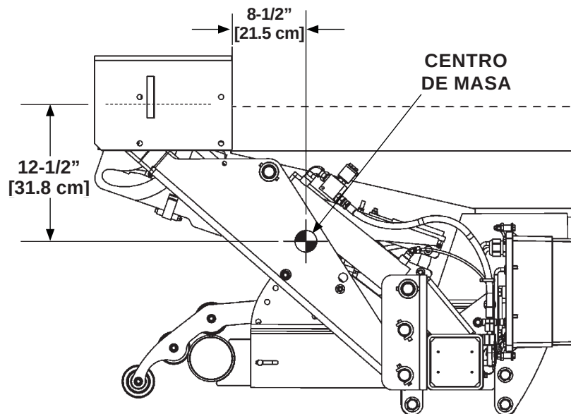
CENTRO DE MASA EN GPTLR-44 Y GPTLR-55 (POSICIÓN DE GUARDADO) FIG. 15-2
