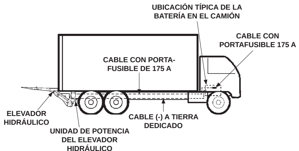
INSTALACIÓN RECOMENDADA PARA EL ELEVADOR Y EL CABLE DE ALIMENTACIÓN EN CAMIONES FIG. 34-2
