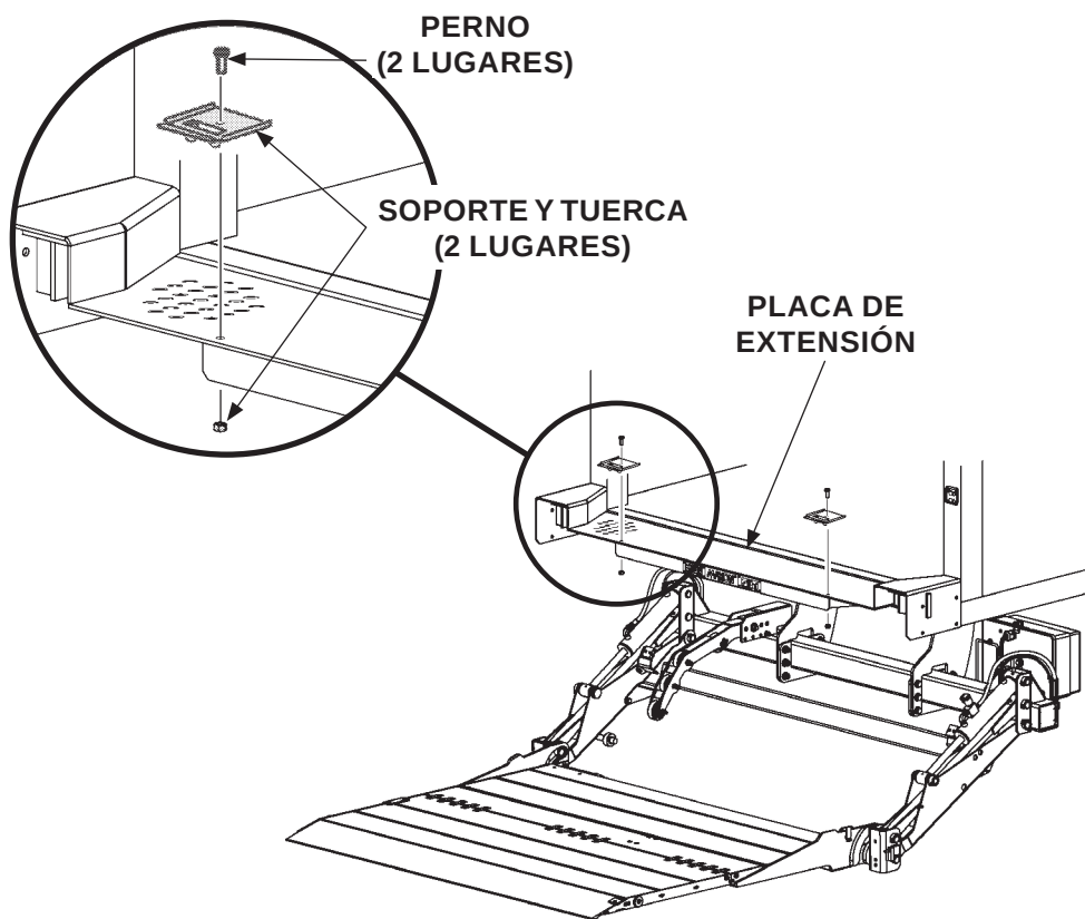
REINSTALACIÓN DE LOS SOPORTES DE INSTALACIÓN FIG. 52-1
