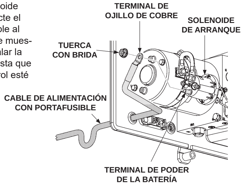
CONECTAR CABLE DE ALIMENTACIÓN CON PORTAFUSIBLE (SE MUESTRA LA BOMBA CON DESCENSO POR GRAVEDAD) FIG. 37-1
