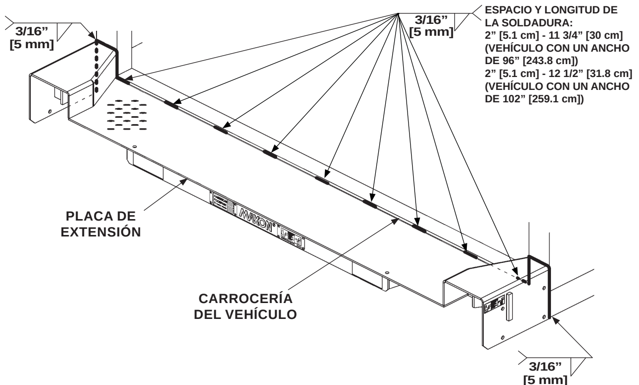
SOLDADURAS DE LA PLACA DE EXTENSIÓN - VISTA DESDE ARRIBA FIG. 19-1
