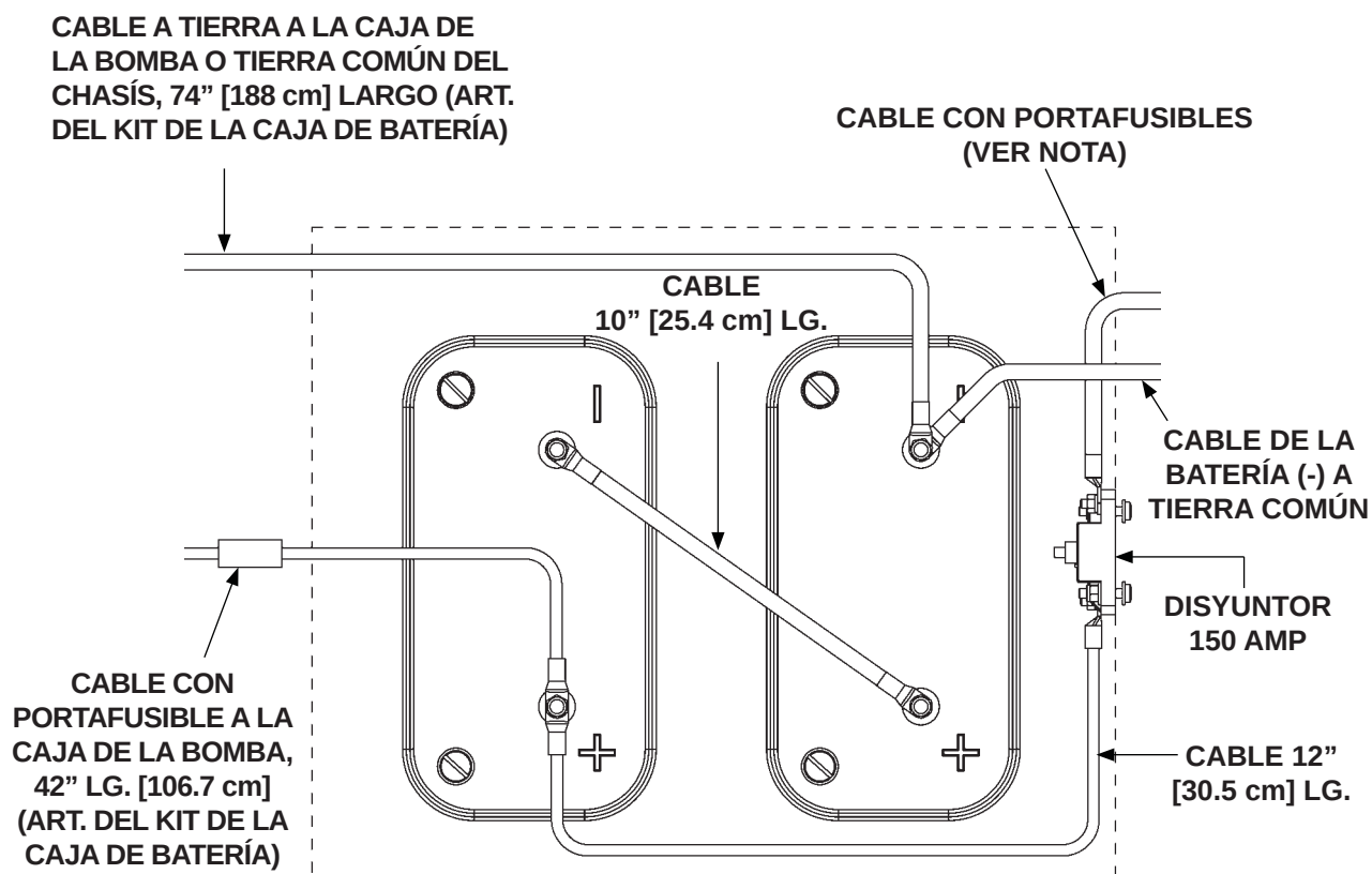
CONEXIONES EN BATERÍA DE 12 V PARA UNA CORRIENTE DE 24 V FIG. 31-1
