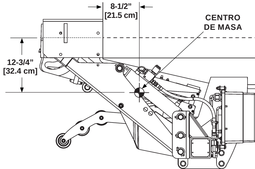
CENTRO DE MASA EN GPTLR-25 Y GPTLR-33 (POSICIÓN DE GUARDADO) FIG. 15-1
