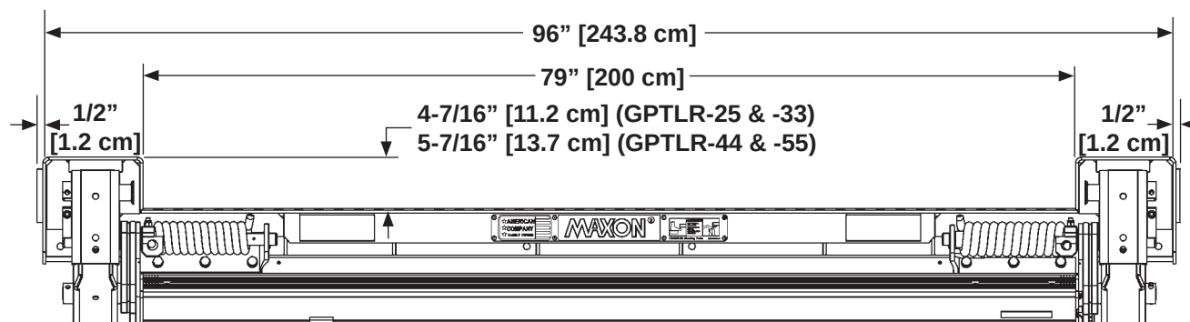
MEDIDAS DE LA PLACA DE EXTENSIÓN PARA GPTLR EN CARROCERÍAS DE 96" [243 cm] DE ANCHO FIG. 12-1
