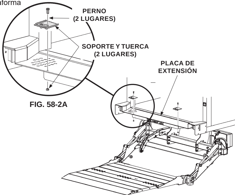
RETIRAR SOPORTES DE INSTALACIÓN FIG. 58-2
