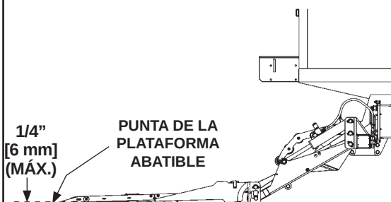
PLATAFORMA Y LOS GRILLETES TOCAN EL SUELO FIG. 49-2
