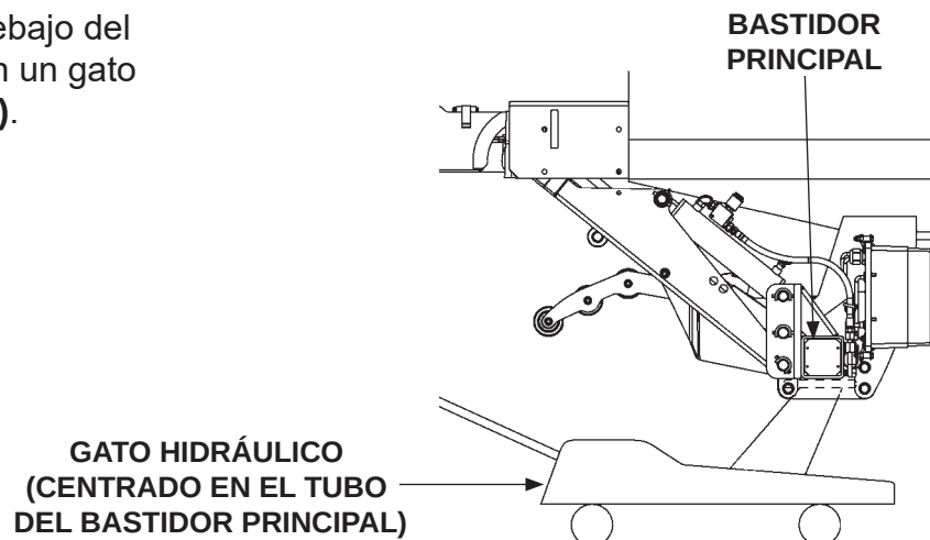
APOYAR EL ELEVADOR HIDRÁULICO FIG. 54-2
