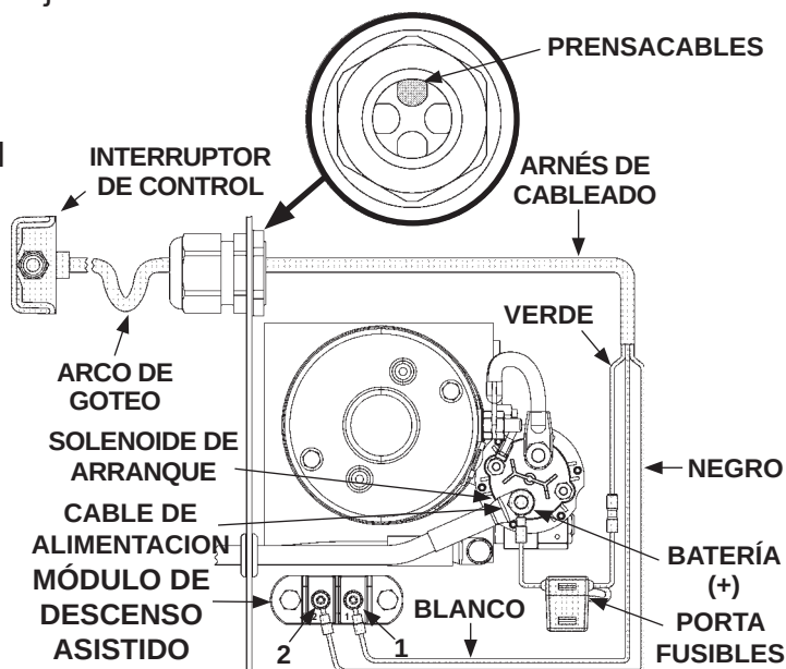
CONEXIONES DE CABLEADO PARA EL INTERRUPTOR DE CONTROL (DESCENSO ASISTIDO) FIG. 41-2
