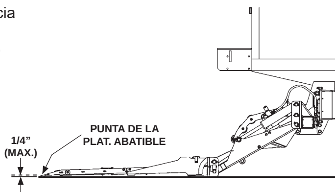
LA PLATAFORMA Y LOS GRILLETES TOCAN EL SUELO FIG. 59-2
