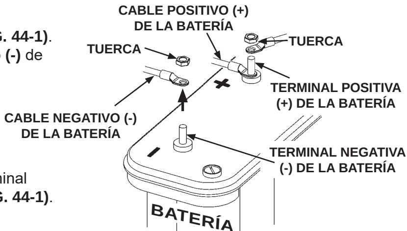
DESCONECTAR EL CABLE NEGATIVO (-) DE LA BATERÍA FIG. 44-1
