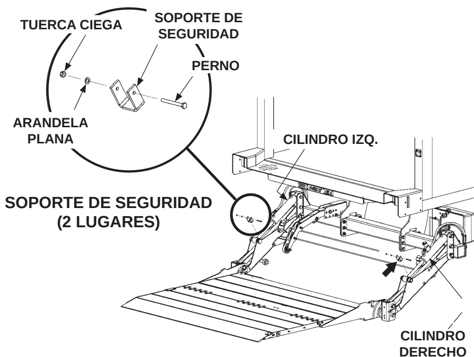
RETIRAR SOPORTES DE SEGURIDAD FIG. 59-1
