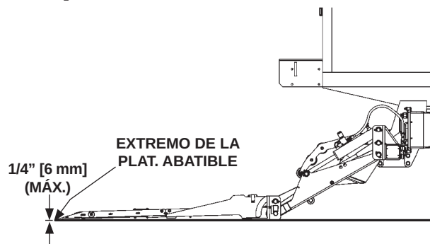
LA PLATAFORMA Y LOS GRILLETES TOCAN EL SUELO FIG. 51-1
