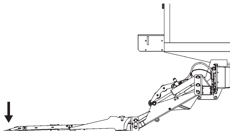
DESCENDER LA PLATAFORMA FIG. 45-2
