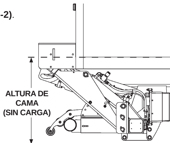
MEDIR LA ALTURA DE CAMA (SE MUESTRA EL DISPOSITIVO DE ANTIEMPOTRAMIENTO ESTÁNDAR) FIG. 66-2
