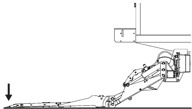
DESCENDER LA PLATAFORMA FIG. 47-2
