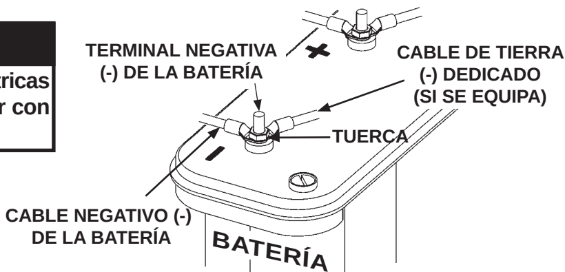
CONECTAR NUEVAMENTE LOS CABLES DE LA BATERÍA FIG. 44-3
