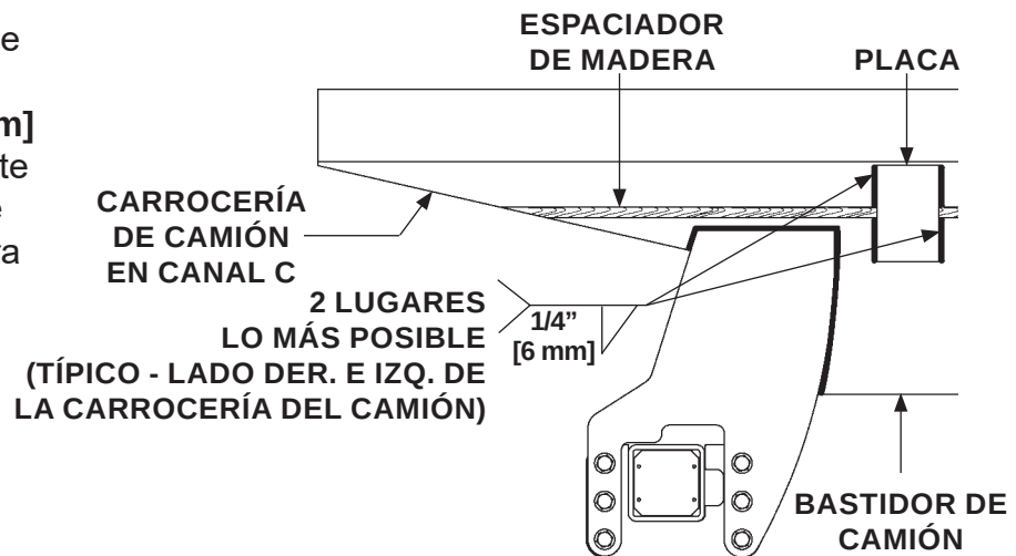
SOLDAR CARROCERÍA DEL CAMIÓN AL BASTIDOR (SE MUESTRA LADO DER.)
