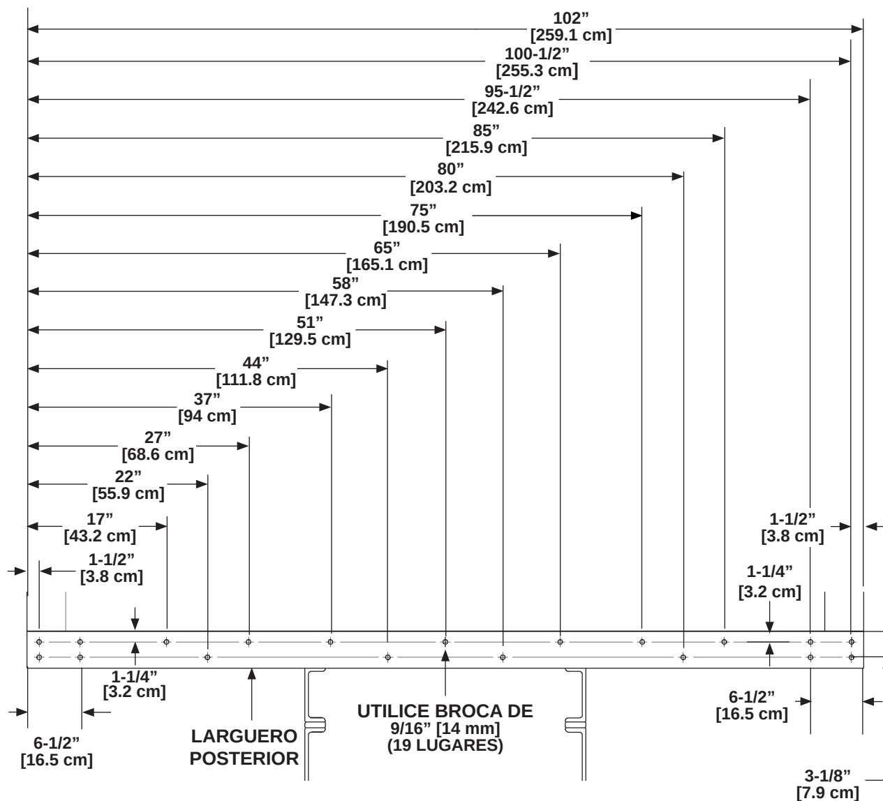
LARGUERO POSTERIOR - UBICACIÓN DE LOS AGUJEROS EN EL VEHÍCULO DE 102" [259.1 cm] DE ANCHO FIG. 17-1
