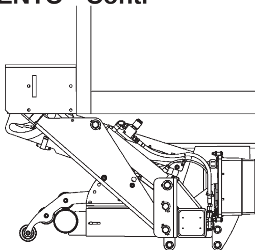
ELEVADOR CON LA PLATAFORMA GUARDADA (SE MUESTRA EL DISPOSITIVO ANTIEMPOTRAMIENTO ESTÁNDAR) FIG. 66-1
