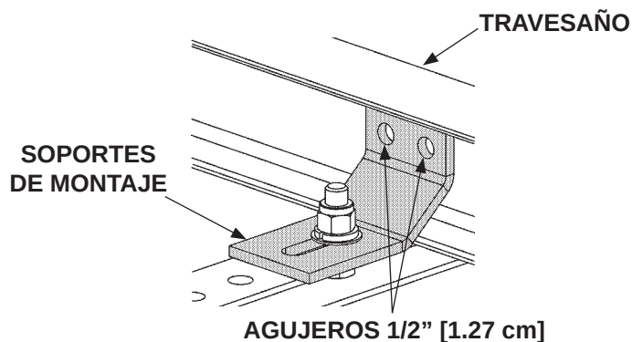
MARCAR Y TALADRAR AGUJEROS PARA LOS SOPORTES FIG. 28-1
