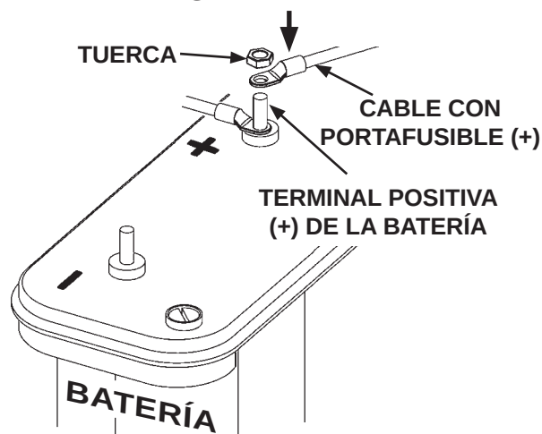
CONECTAR EL CABLE CON PORTAFUSIBLE (+) FIG. 44-2
