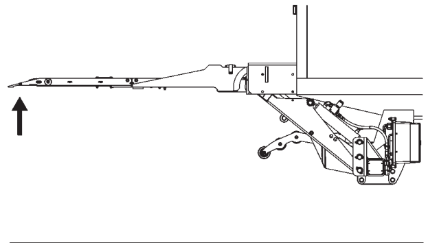
ELEVAR LA PLATAFORMA FIG. 47-3
