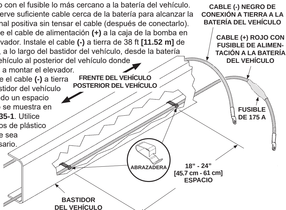
INSTALACIÓN DE CABLES DE ALIMENTACIÓN Y CONEXIÓN A TIERRA AL ELEVADOR EN EL CAMIÓN FIG. 35-1
