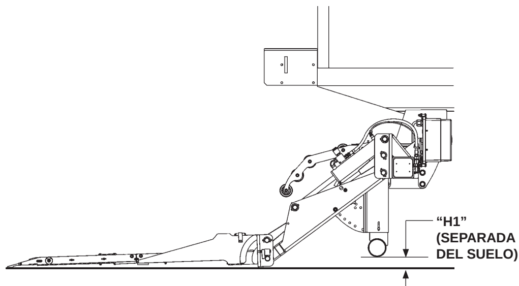
ANTIEMPOTRAMIENTO FMVSS ESTÁNDAR FIG. 73-2
