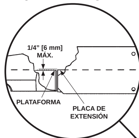
ESPACIO VERTICAL FIG. 49-1A
