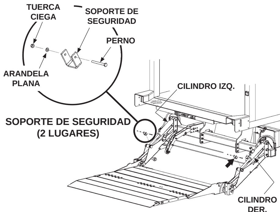
REINSTALAR LOS SOPORTES DE SEGURIDAD FIG. 53-1
