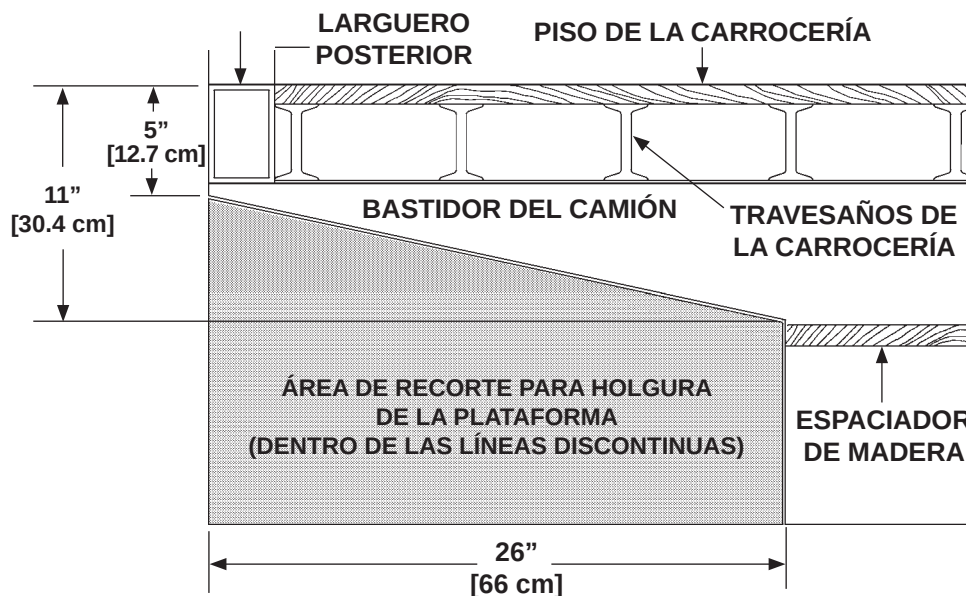
CORTE DEL BASTIDOR DEL VEHÍCULO PARA TODOS LOS MODELOS GPTLR
