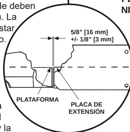
ESPACIO HORIZONTAL FIG. 49-1B
