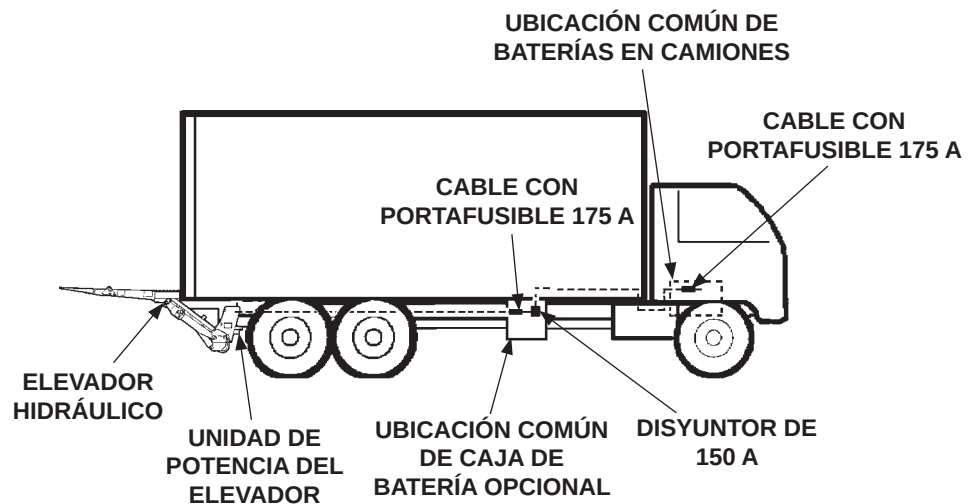
INSTALACIÓN RECOMENDADA DEL ELEVADOR Y DE LA CAJA DE BATERÍAS EN CAMIONES
