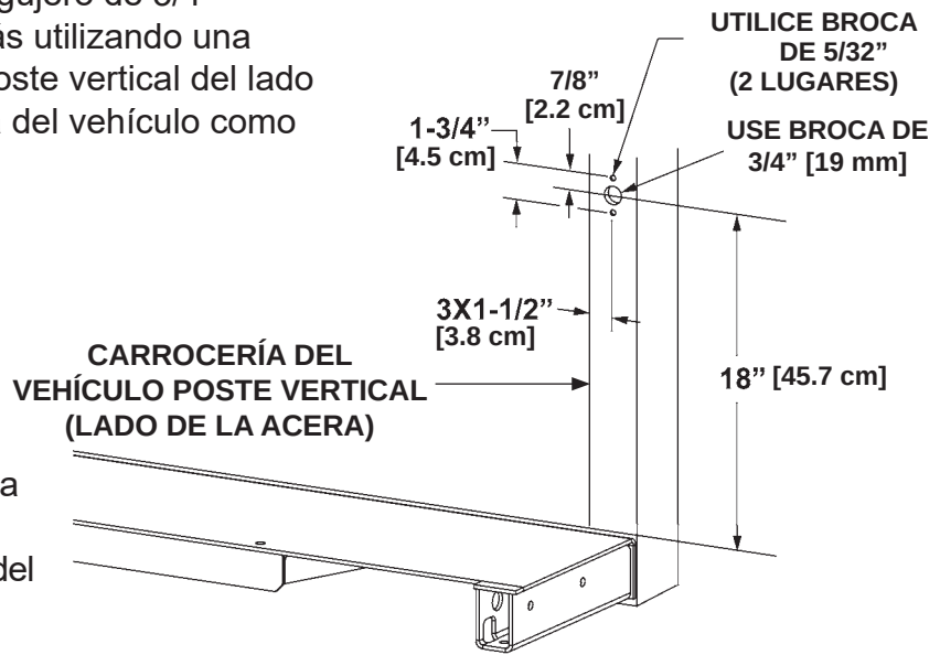
TALADRAR ORIFICIOS PARA MONTAJE FIG. 40-1
