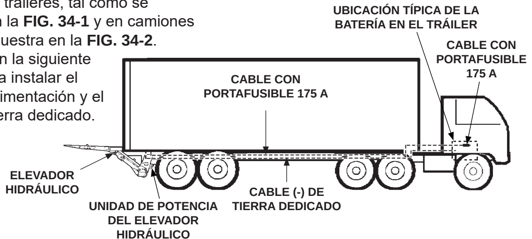
INSTALACIÓN RECOMENDADA PARA EL ELEVADOR Y EL CABLE DE ALIMENTACIÓN EN TRÁILER FIG. 34-1
