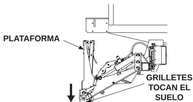
PLATAFORMA DESCENDIDA DESDE LA POSICIÓN REPLEGADA (SE MUESTRA LADO DERECHO)
