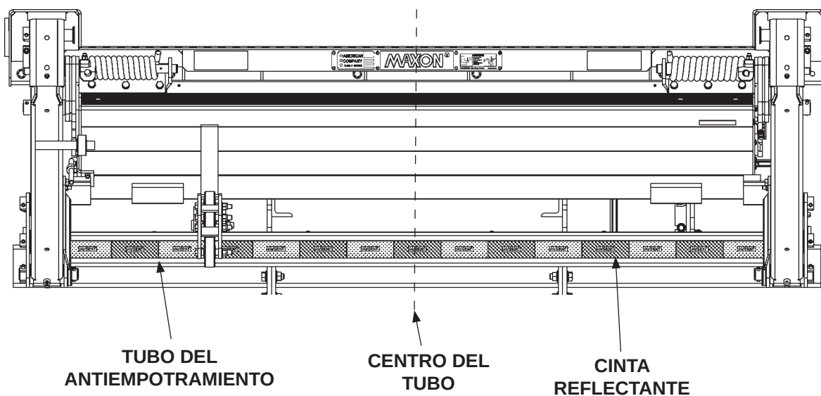
AÑADIR LA CINTA REFLECTANTE FIG. 78-1
