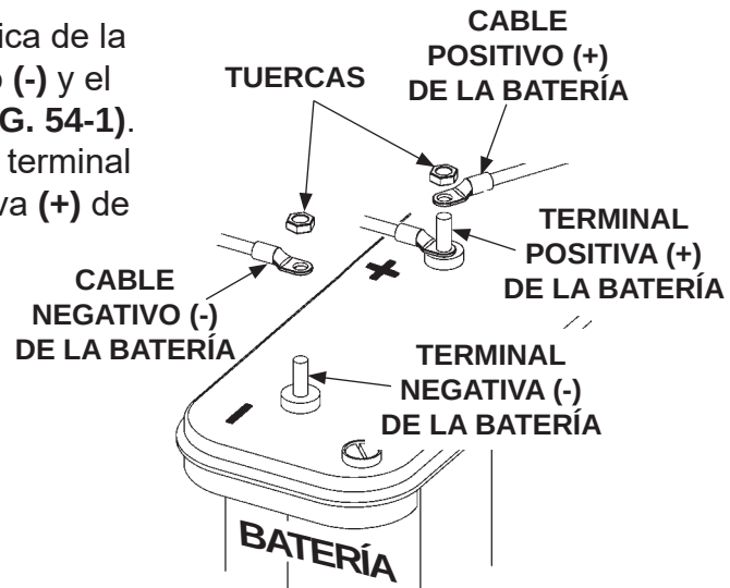
DESCONECTAR LA ALIMENTACIÓN ELÉCTRICA DE LA BATERÍA FIG. 54-1
