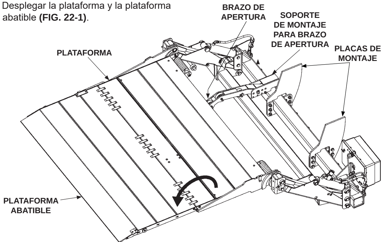
PLATAFORMA Y PLATAFORMA ABATIBLE FIG. 22-1
