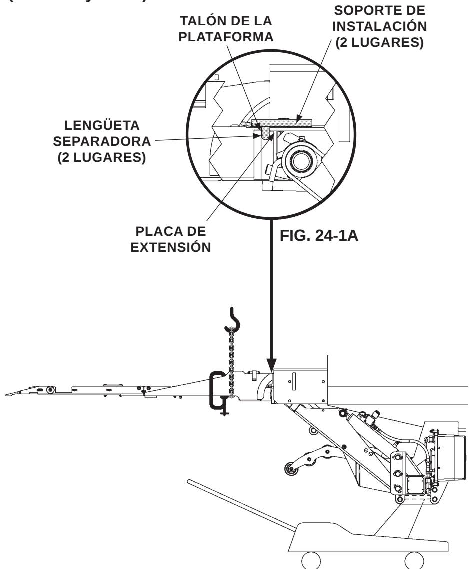
PLATAFORMA AJUSTADA FIRMEMENTE CONTRA LAS LENGÜETAS DEL SOPORTE DE INSTALACIÓN FIG. 24-1
