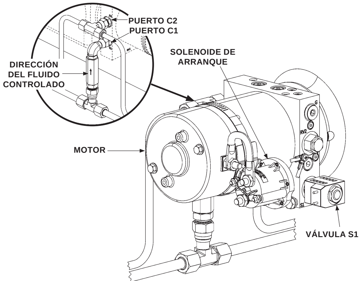
UNIDAD DE POTENCIA CON DESCENSO ASISTIDO FIG. 85-1
