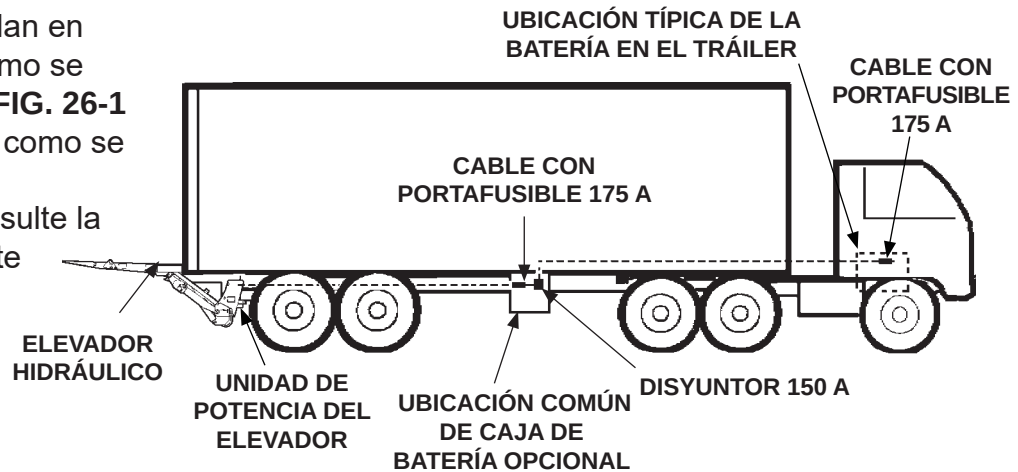
INSTALACIÓN RECOMENDADA DEL ELEVADOR Y DE LA CAJA DE BATERÍAS OPCIONAL EN TRÁILER
