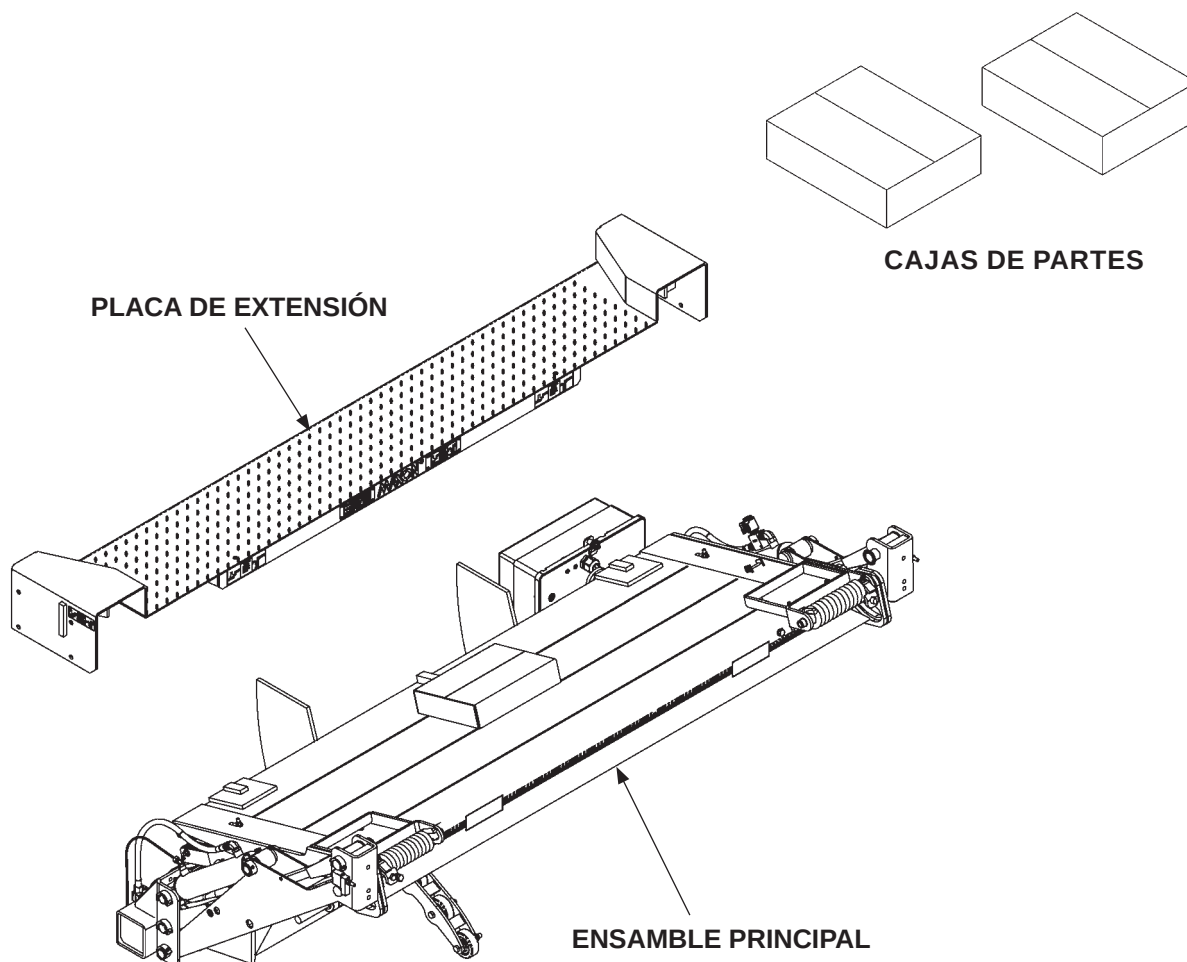
COMPONENTES DEL GPTLR FIG. 7-1
