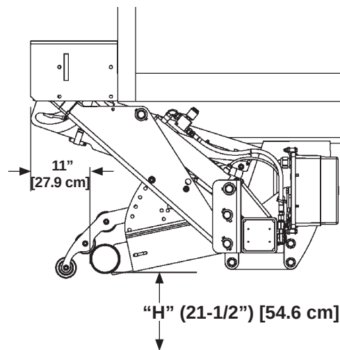
ANTIEMPOTRAMIENTO FMVSS ESTÁNDAR FIG. 73-1
