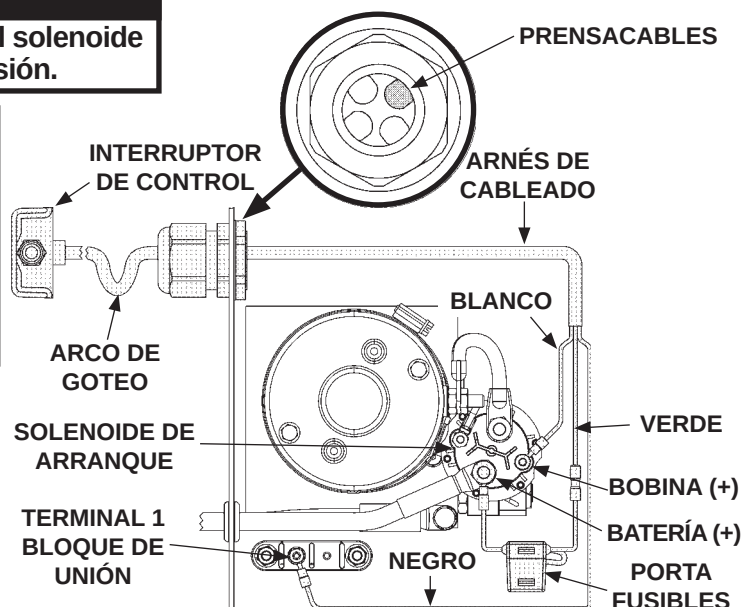
CONEXIONES DE CABLEADO PARA EL INTERRUPTOR DE CONTROL (DESCENSO POR GRAVEDAD) FIG. 41-1
