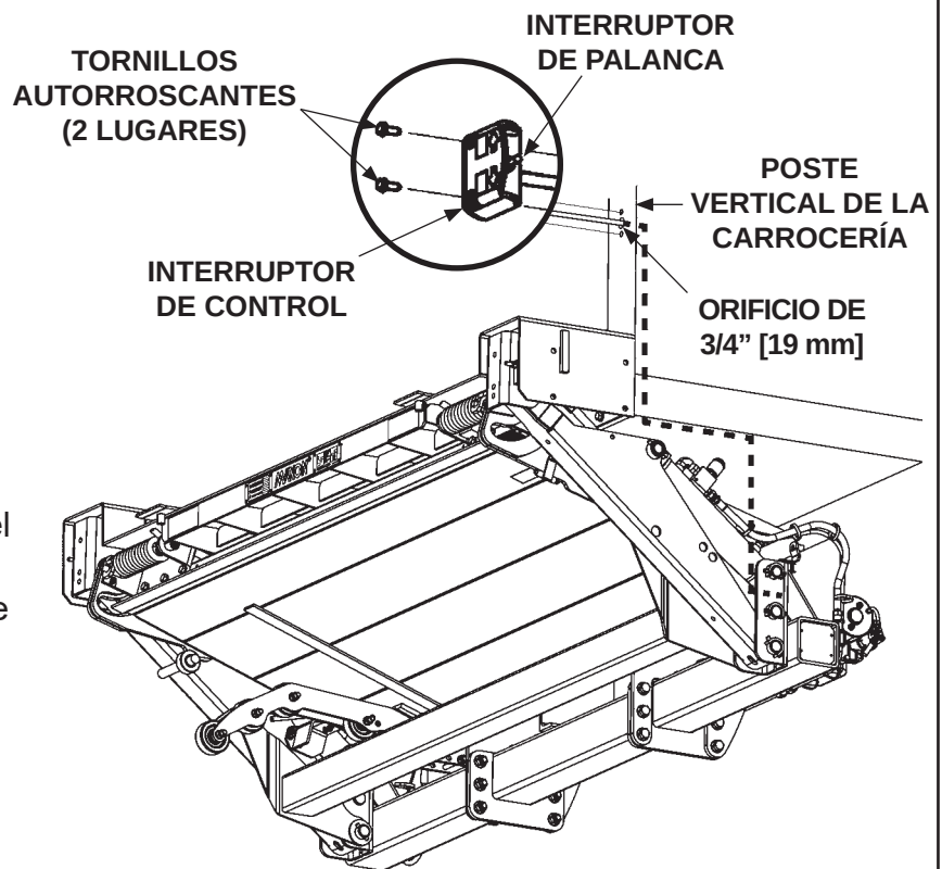
ENRUTAMIENTO DE CABLEADO DEL INTERRUPTOR DE CONTROL FIG. 40-2
