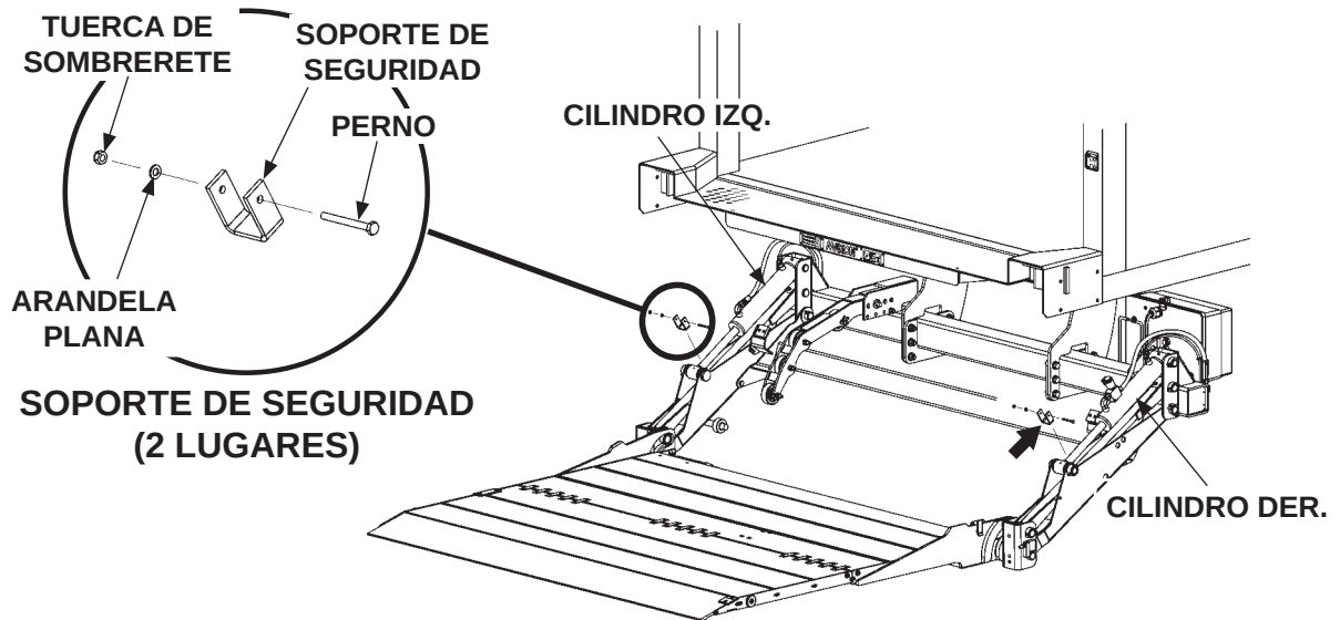
RETIRAR LOS SOPORTES DE SEGURIDAD FIG. 46-1
