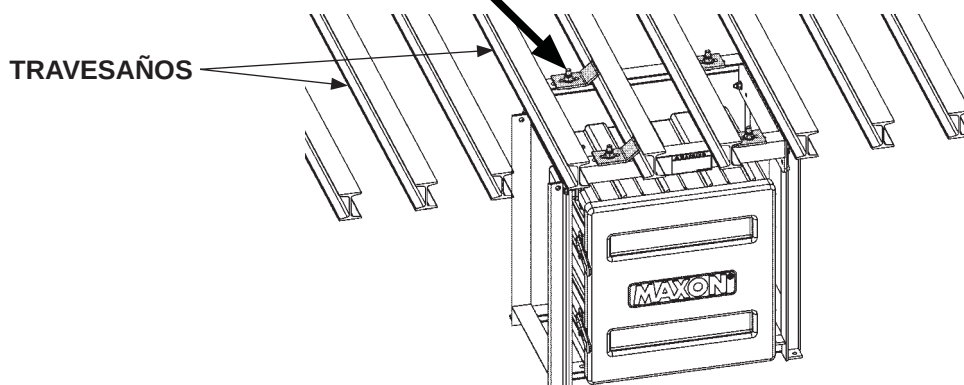
ATORNILLAR EL BASTIDOR DE LA CAJA DE LA BATERÍA FIG. 28-2
