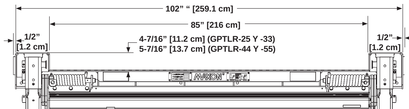
MEDIDAS DE LA PLACA DE EXTENSIÓN PARA GPTLR PARA CARROCERÍAS DE 102" [259 cm] DE ANCHO FIG. 12-2
