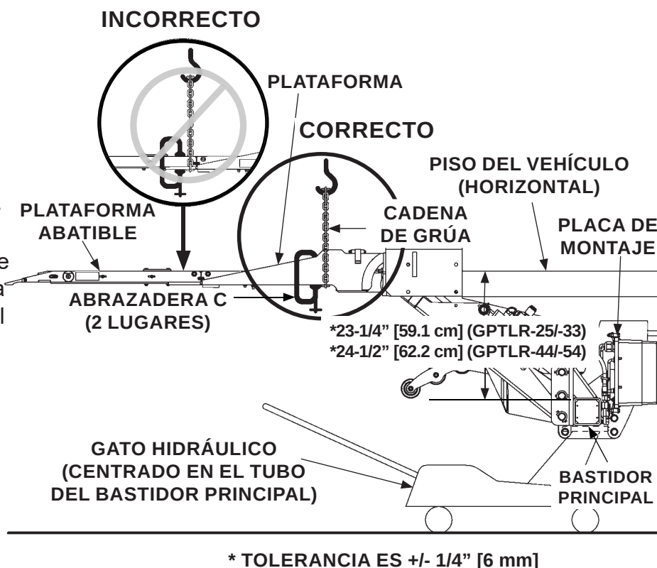
MANERA CORRECTA DE LEVANTAR EL ELEVADOR CON UNA GRÚA FIG. 55-1
