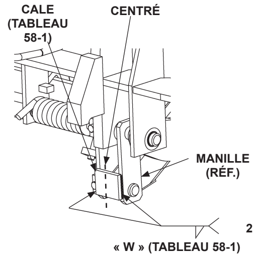
SOUDEGE DE LA CALE (MANILLE DROITE INDIQUÉE) FIG. 59-2
