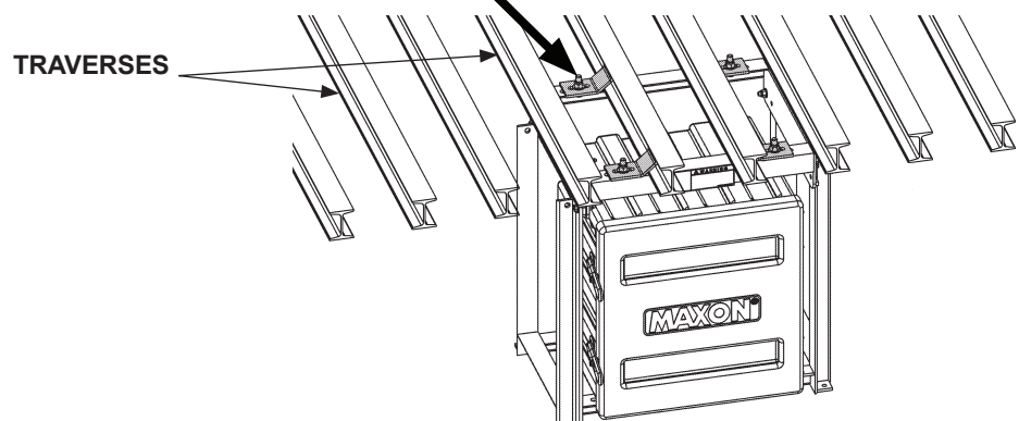
BOULONNER LE CADRE DU BOÎTIER DE LA BATTERIE FIG. 33-2
