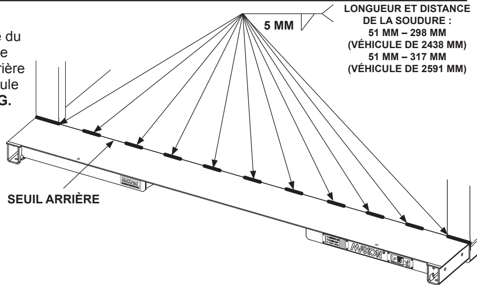
SOUDURES DE LA PLAQUE DE RALLONGE – VUES DE DESSUS FIG. 18-1
