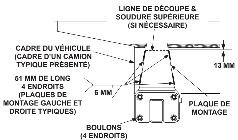
TE-20 SOUDER AU CADRE DU VÉHICULE (CÔTÉ DROIT MONTRÉ) FIG. 30-1
