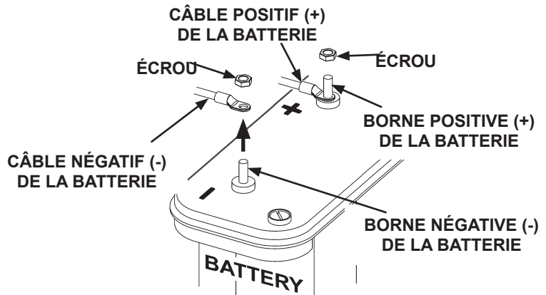
DÉCONNEXION DU (-) CÂBLE DE LA BATTERIE FIG. 50-1
