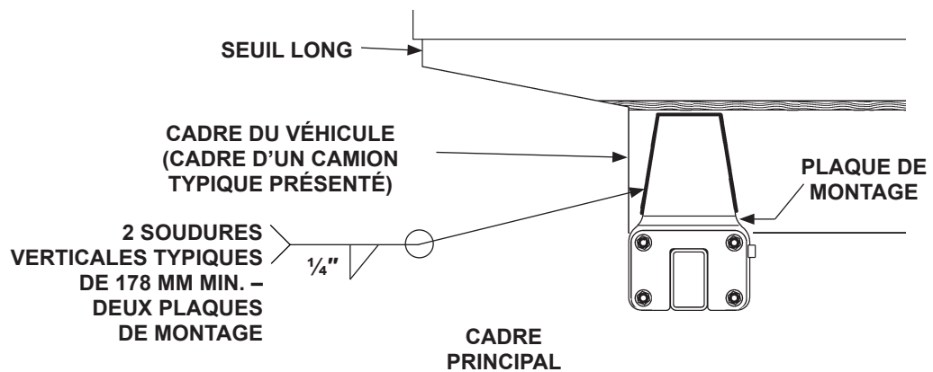
TE-20 PLAQUE DE MONTAGE SOUDÉE AU CHÂSSIS DU CAMION & BOULONNÉE AU CHÂSSIS PRINCIPAL FIG. 61-2
