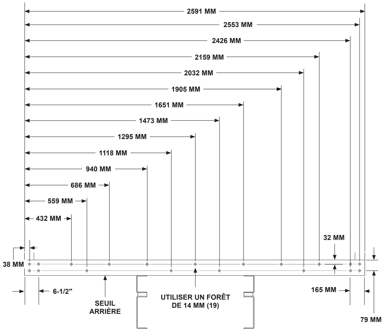
SEUIL ARRIÈRE – EMPLACEMENT DES TROUS POUR UN VÉHICULE DE 2591 MM DE LARGE FIG. 21-1
