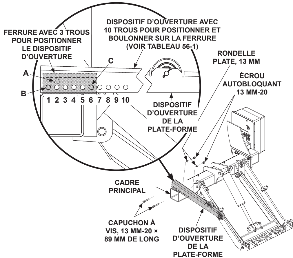
BOULONNER LE DISPOSITIF D'OUVERTURE DE LA PLATE-FORME (SÉRIE TE) FIG. 55-1
