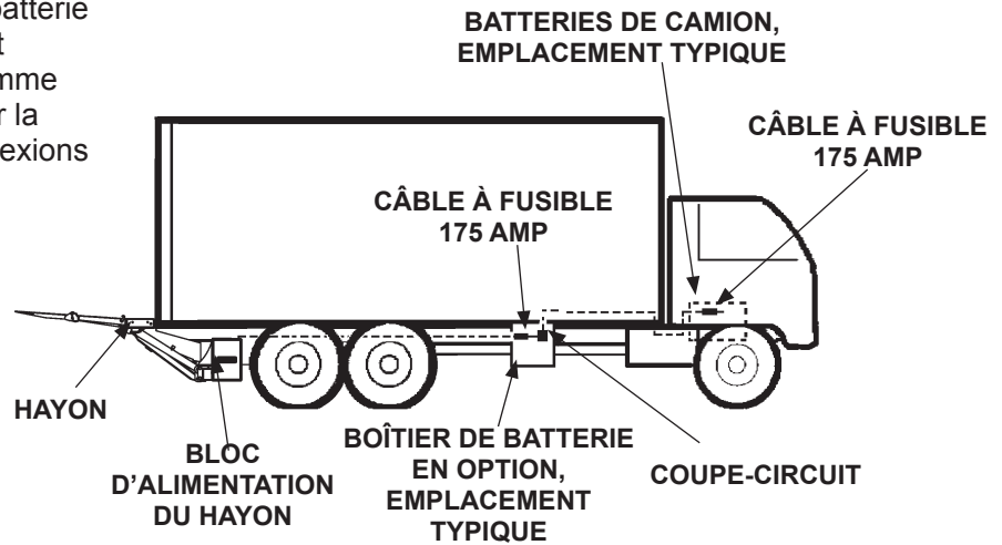
RECOMMANDATION POUR L'INSTALLATION DU HAYON ET DU BOÎTIER DE BATTERIE SUR LE CAMION FIG. 31-1
