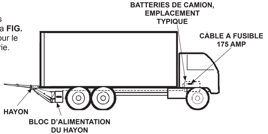
RECOMMANDATION POUR L'INSTALLATION DU HAYON ET DU BOÎTIER DE BATTERIE SUR LE CAMION FIG. 39-1
