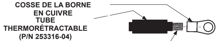
PLACEMENT DE LA COSSE DE LA BORNE & D'UN TUBE THERMORÉTRACTABLE SUR UN CÂBLE D'ALIMENTATION À FUSIBLE FIG. 42-1
