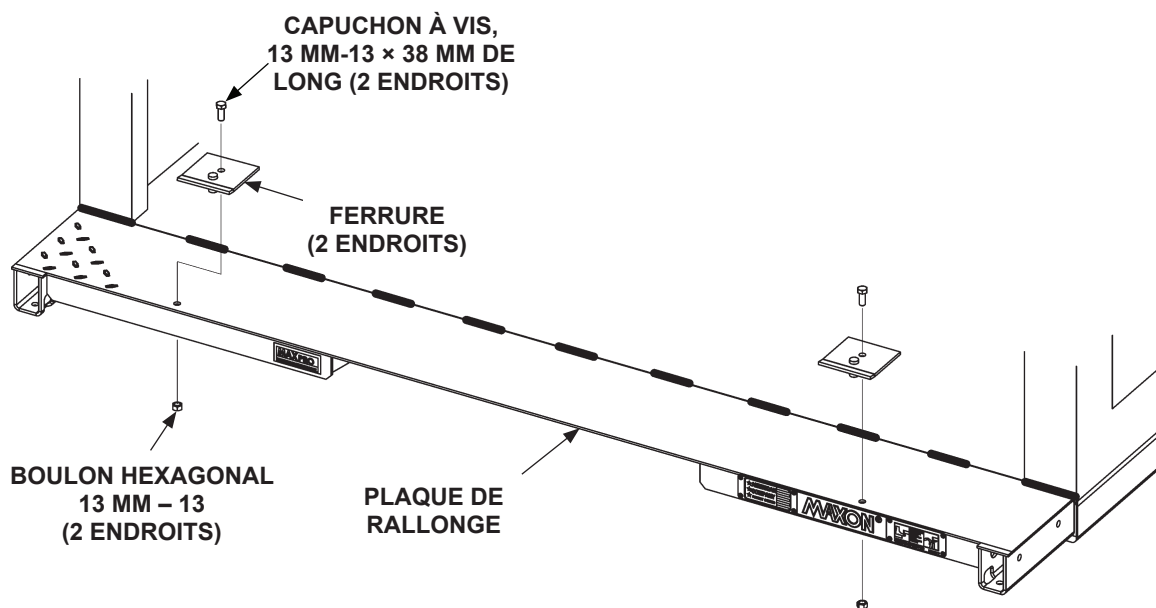
BOULONNAGE SUR LES FERRURES D'INSTALLATION FIG. 23-1
