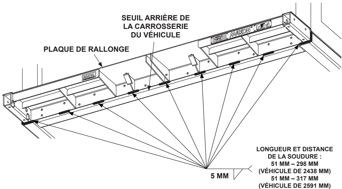
SOUDURES DE LA PLAQUE DE RALLONGE – VUES DE DESSOUS FIG. 19-2
