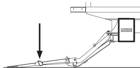
BAISSER LA PLATE-FORME FIG. 52-2
