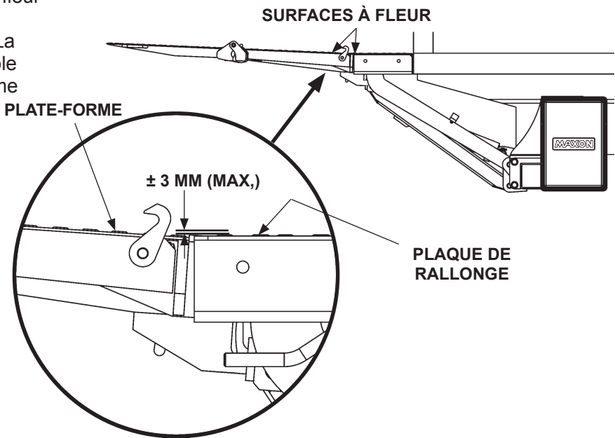
DIFFÉRENCE MAXIMALE DE HAUTEUR POUR LE HAUT DE LA PLATE-FORME & LA PLAQUE DE RALLONGE (VUE DE DROITE) FIG. 54-1
