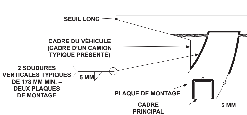
TE-25 & TE-30 PLAQUE DE MONTAGE SOUDÉE AU CHÂSSIS DU CAMION & AU CHÂSSIS PRINCIPAL FIG. 62-1
