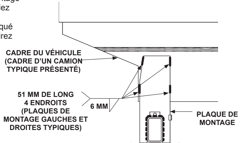
TE-20 SOUDER AU CADRE DU VÉHICULE (CÔTÉ DROIT MONTRÉ) FIG. 29-1
