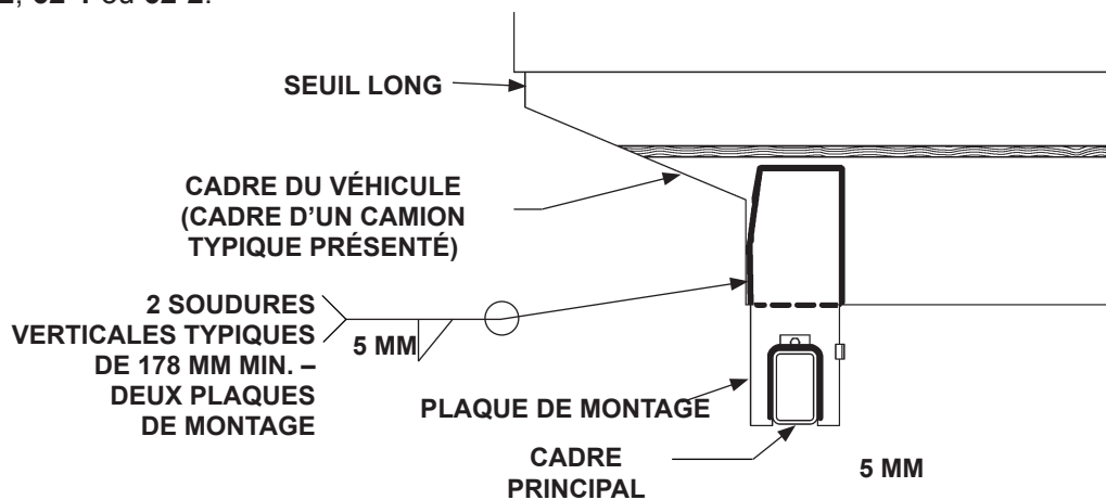
TE-20 PLAQUE DE MONTAGE SOUDÉE AU CHÂSSIS DU CAMION & AU CHÂSSIS PRINCIPAL FIG. 61-1
