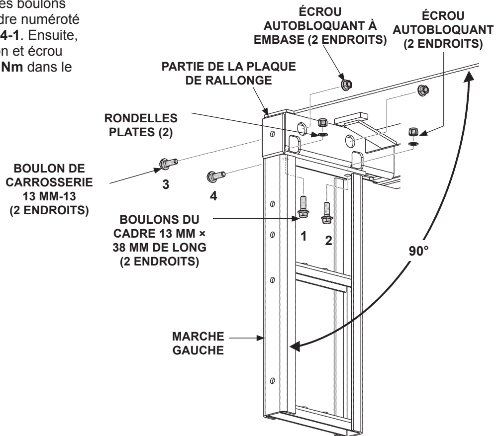
BOULONNER LA MARCHE À LA PLAQUE DE RALLONGE (MARCHE DOUBLE GAUCHE INDIQUÉE) FIG. 64-1
