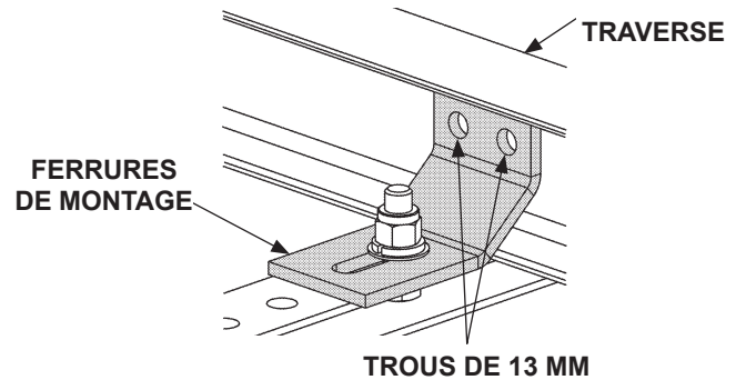
MARQUER ET PERCER DES TROUS DANS LES FERRURES FIG. 33-1
