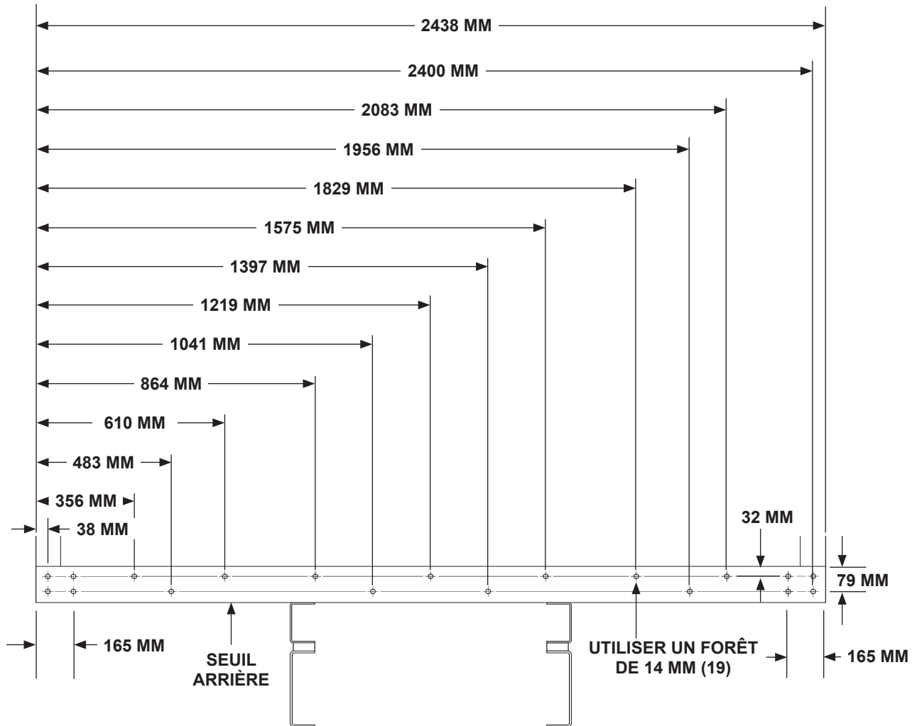
SEUIL ARRIÈRE – EMPLACEMENT DES TROUS POUR UN VÉHICULE DE 2439 MM DE LARGE FIG. 20-1
