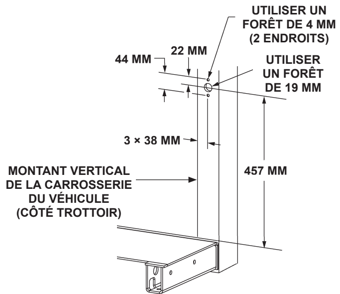
PERÇAGE DES TROUS DE MONTAGE FIG. 45-1
