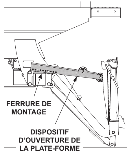
CONTRÔLER LA POSITION DU DISPOSITIF D'OUVERTURE FIG. 57-1
