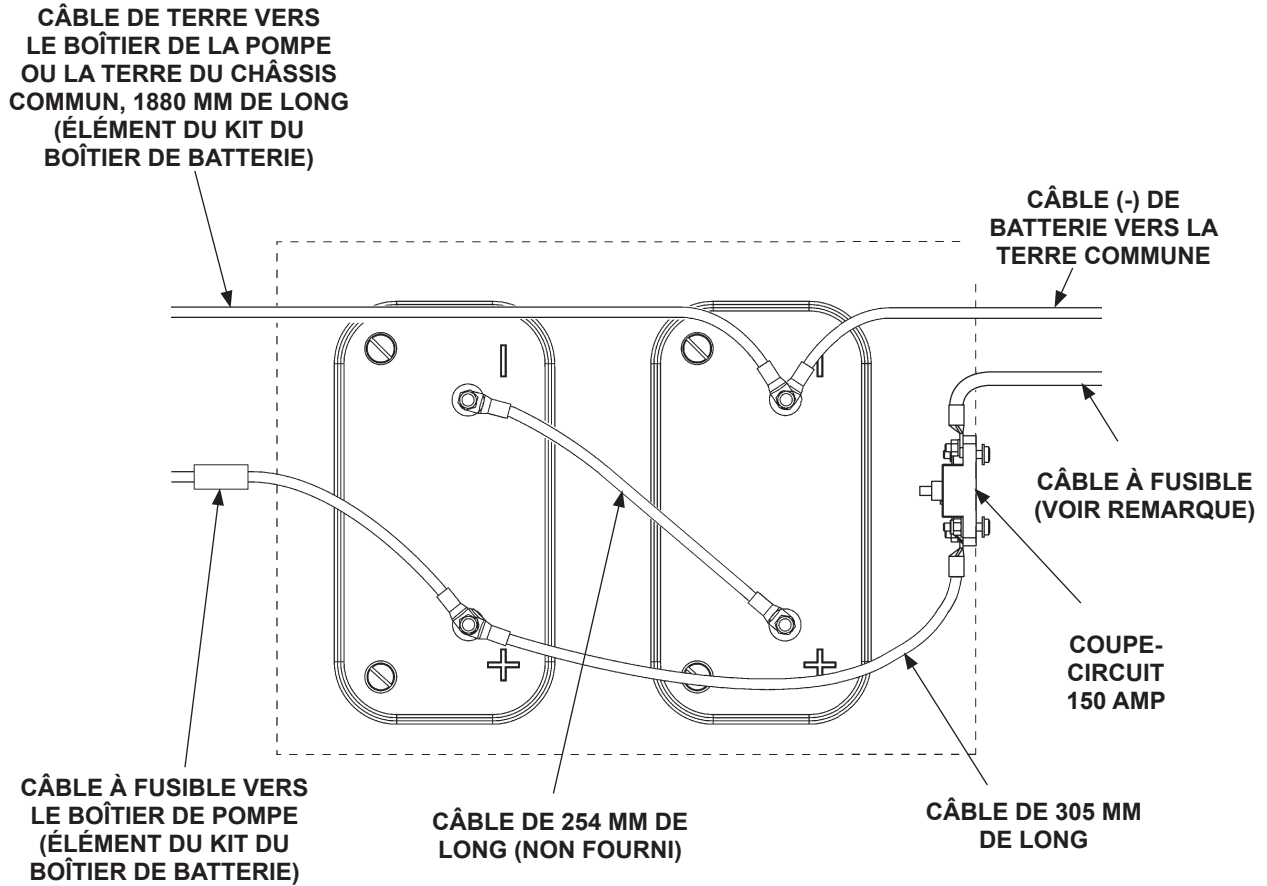
CONNEXIONS DE BATTERIE 12 VOLTS POUR UNE PUISSANCE DE 24 VOLTS FIG. 36-1
