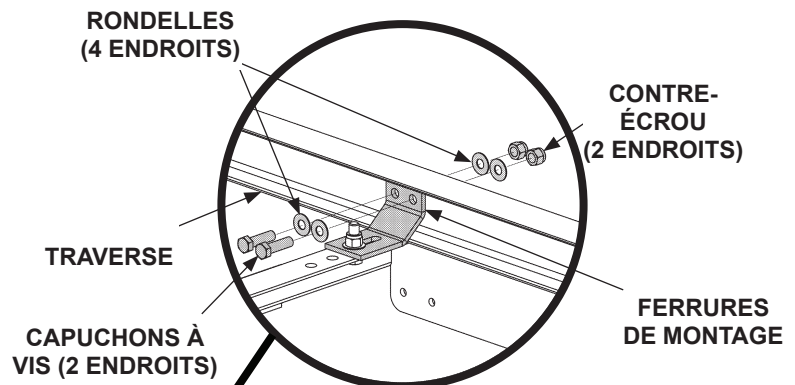
MARQUER ET PERCER DES TROUS DANS LES FERRURES FIG. 33-1
