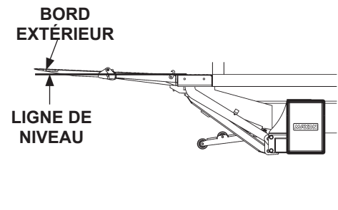
BORD DE LA PLATE-FORME AU-DESSUS DU PLANCHER FIG. 58-2
