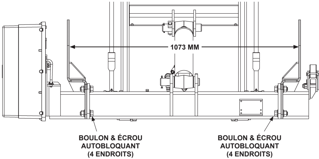
PLAQUES DE MONTAGE BOULONNÉES À 1073 MM (GALVANISÉES) FIG. 25-1
