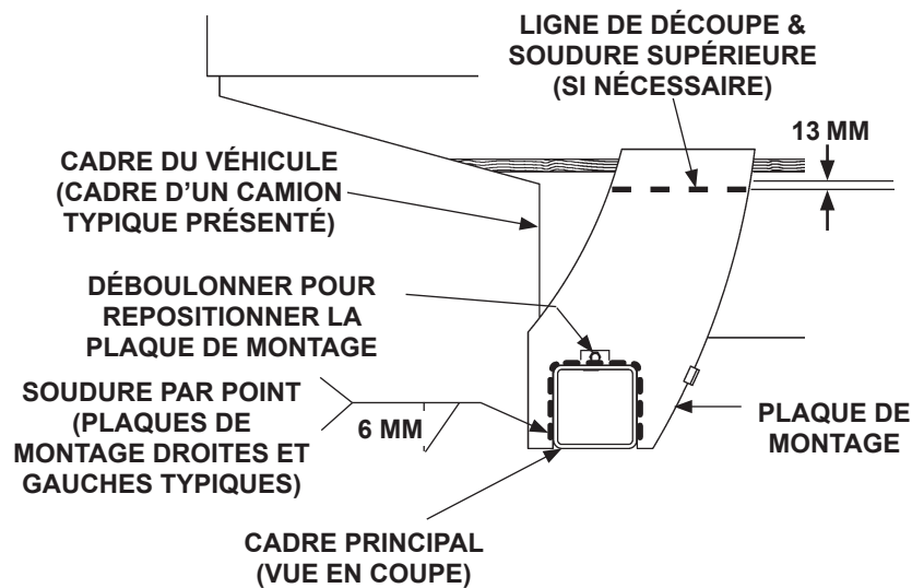
TE-25 & TE-30 REPOSITIONNEMENT DE LA PLAQUE DE MONTAGE PEINTE (CÔTÉ DROIT REPRÉSENTÉ) FIG. 28-2
