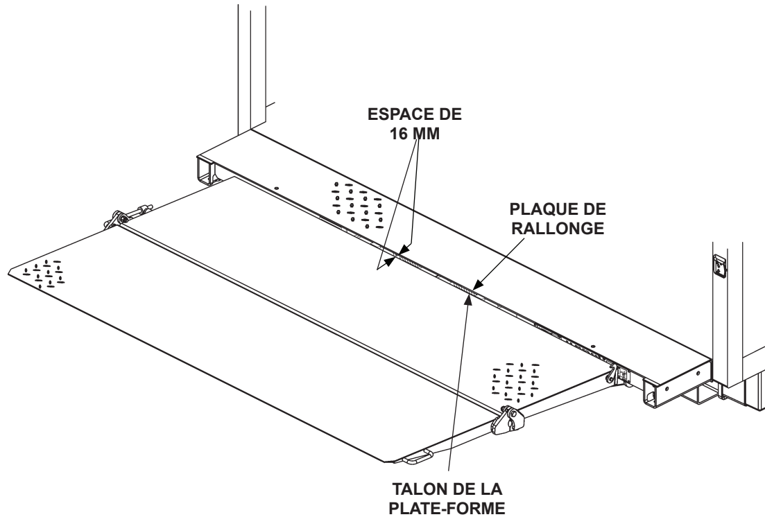
PLATE-FORME À NIVEAU DE PLANCHER AVEC UN ESPACE DE 16 MM ENTRE LE TALON ET LA PLAQUE DE RALLONGE FIG. 53-1
