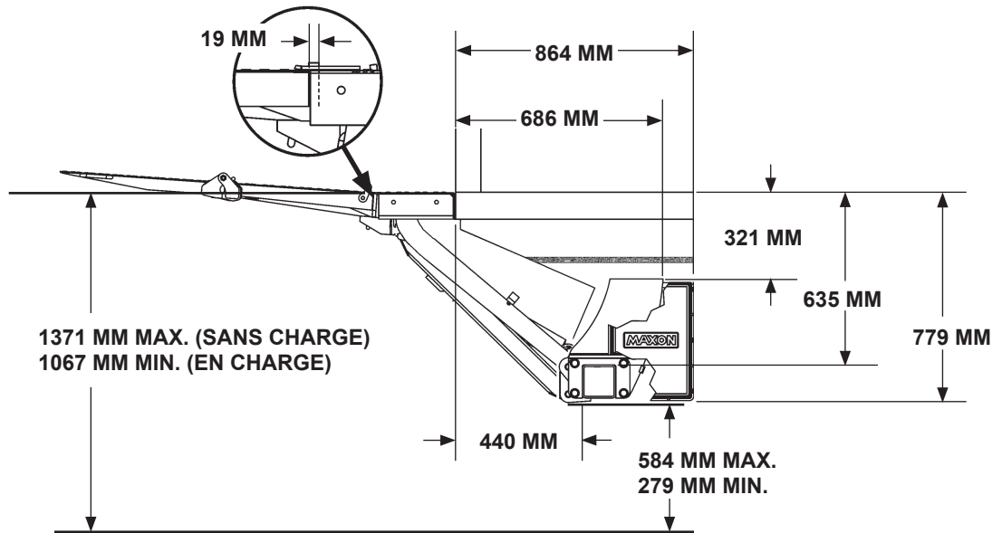
DÉGAGEMENTS POUR UNE INSTALLATION TE-25 & TE-30 À PLANCHER HAUT FIG. 14-1
