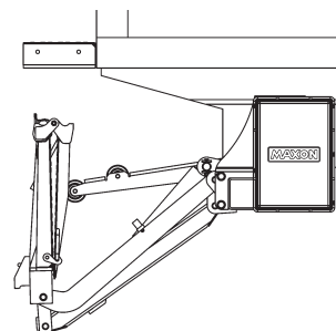
PLATE-FORME SORTIE FIG. 57-3
