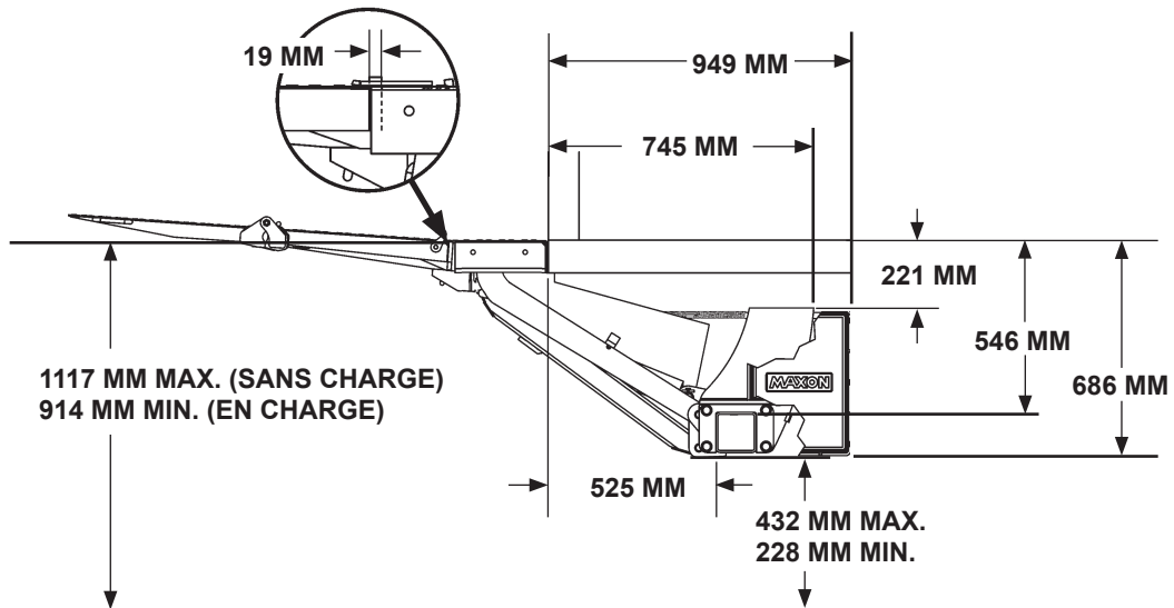
DÉGAGEMENTS POUR UNE INSTALLATION TE-25 & TE-30 À PLANCHER BAS FIG. 14-2
