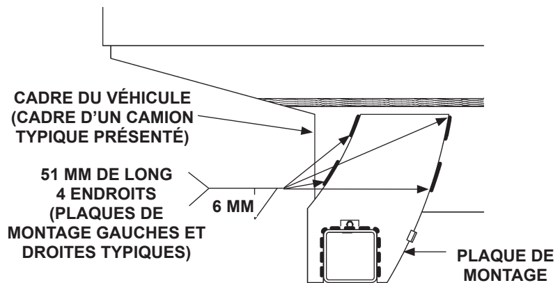
TE-25 & TE-30 SOUDER AU CADRE DU VÉHICULE ET AU CADRE PRINCIPAL (CÔTÉ DROIT MONTRÉ) FIG. 29-2
