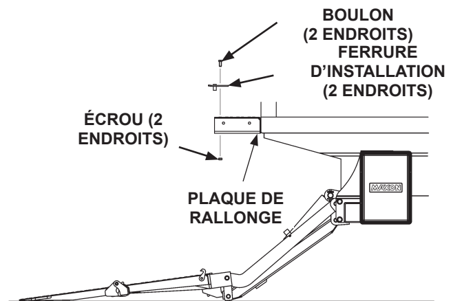
RETRAIT DES FERRURES D'INSTALLATION FIG. 52-4
