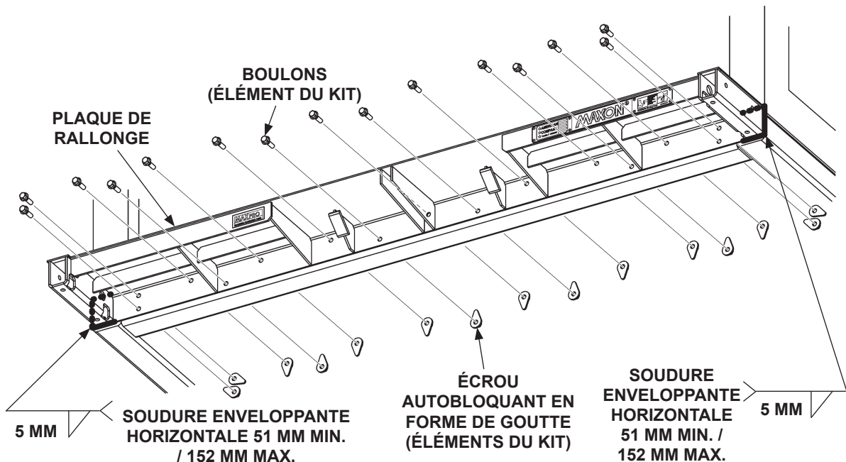
BOULONNER LA PLAQUE DE RALLONGE (PLAQUE DE RALLONGE DE 2438 MM PRÉSENTÉE) FIG. 22-1
