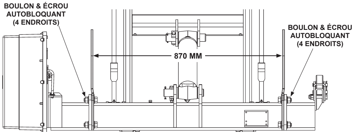
PLAQUES DE MONTAGE BOULONNÉES À 870 MM (GALVANISÉES) FIG. 24-1
