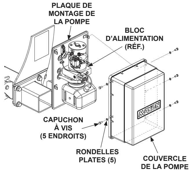
DÉBOULONNAGE DU COUVERCLE DE POMPE FIG. 41-1
