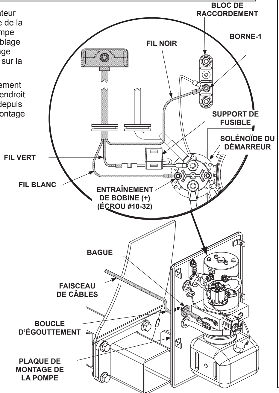
COMMUTATEUR DE COMMANDE CONNECTÉ À L'ASSEMBLAGE DE LA POMPE À DESCENTE PAR GRAVITÉ FIG. 46-1
