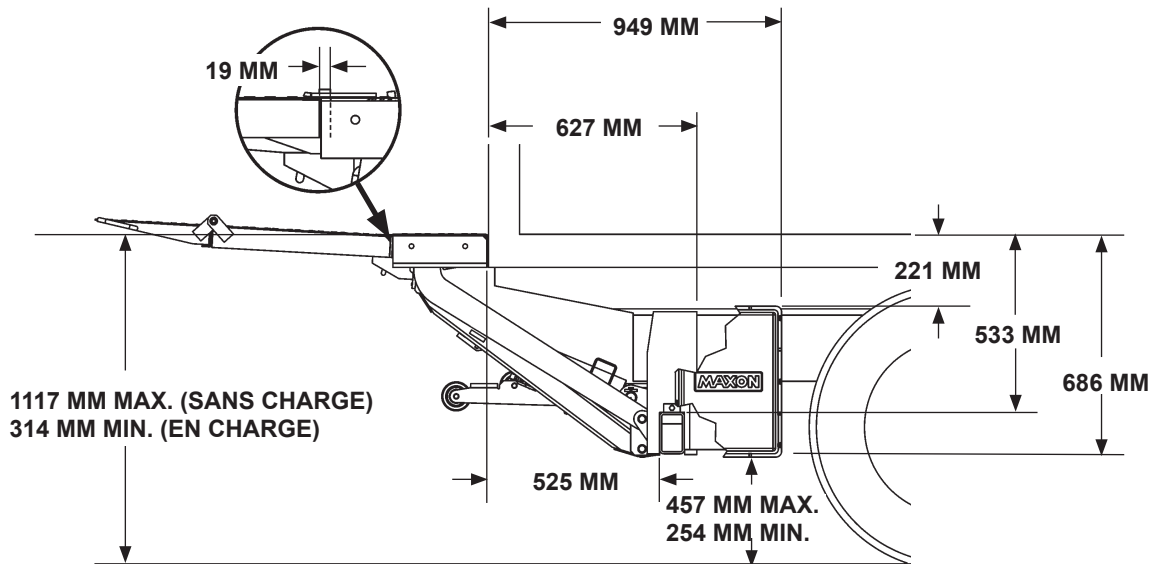
DÉGAGEMENTS POUR UNE INSTALLATION TE-20 À PLANCHER BAS (PEINTE) FIG. 12-2
