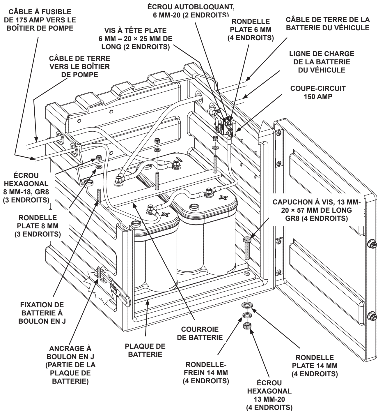
ASSEMBLAGE DU BOÎTIER DE LA BATTERIE (CONNEXION 12 VOLTS MONTRÉE) FIG. 38-1
