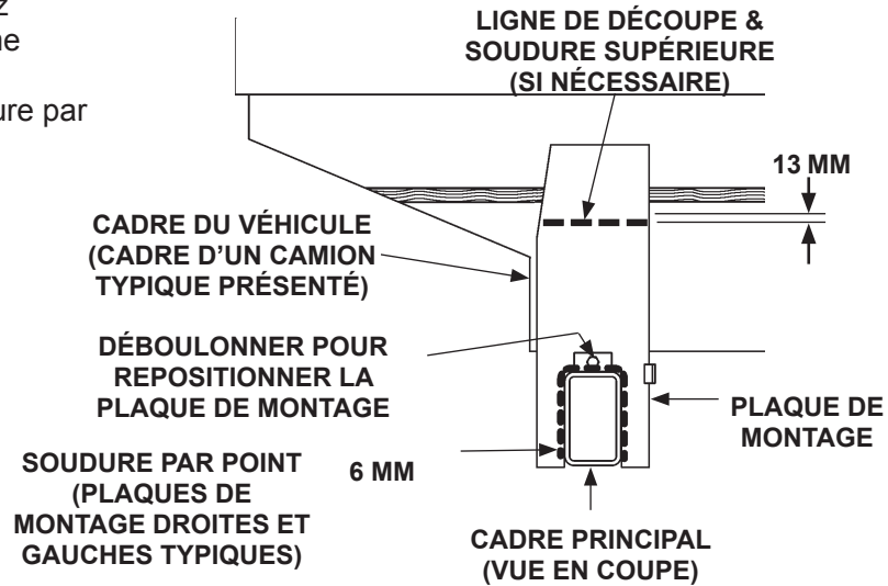
TE-20 REPOSITIONNEMENT DE LA PLAQUE DE MONTAGE PEINTE (CÔTÉ DROIT REPRÉSENTÉ) FIG. 28-1
