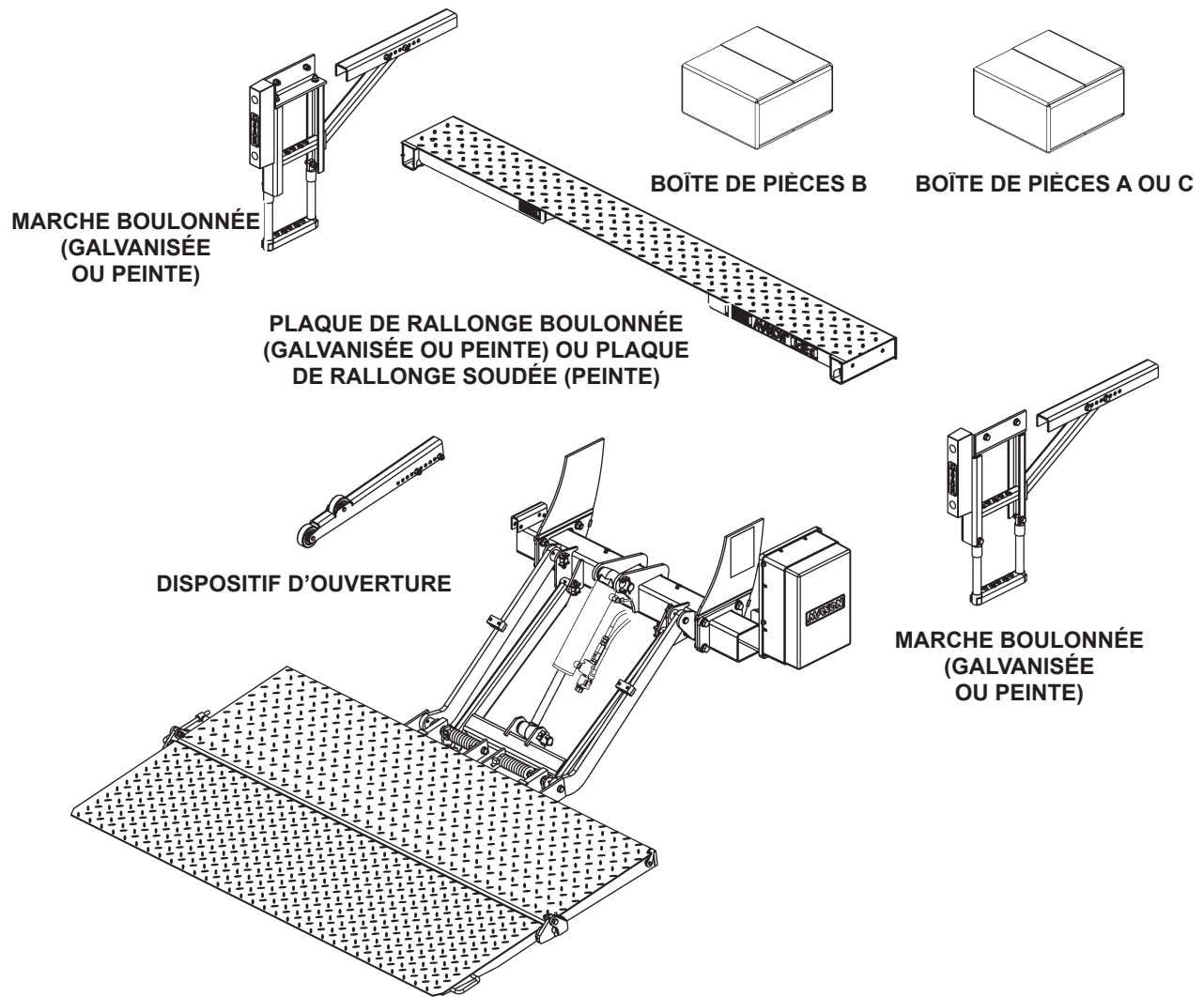
COMPOSANTS DU HAYON FIG. 7-1
