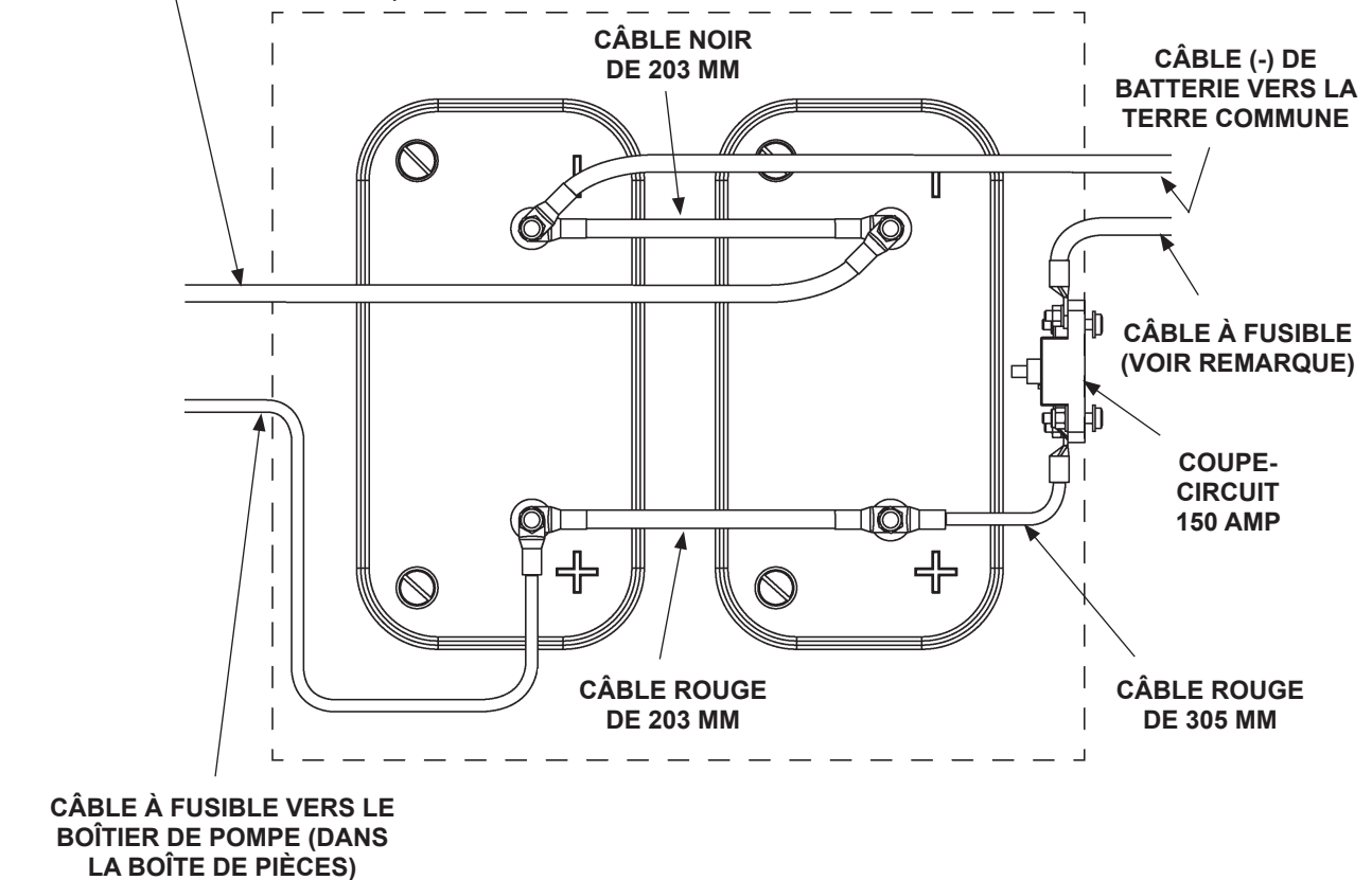
CONNEXIONS DE BATTERIE 12 VOLTS POUR UNE PUISSANCE DE 12 VOLTS FIG. 35-1
