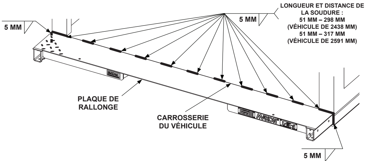
SOUDURES DE LA PLAQUE DE RALLONGE – VUES DE DESSUS FIG. 19-1
