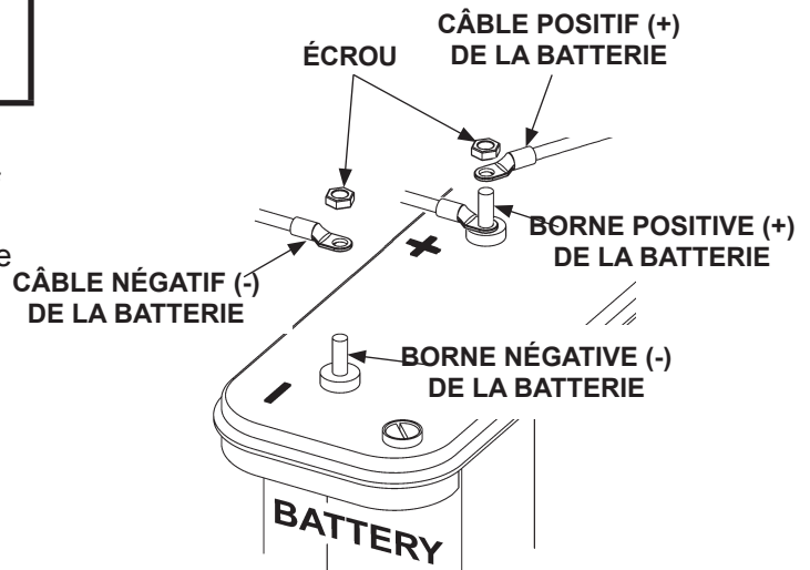
DÉCONNECTER L'ALIMENTATION DE LA BATTERIE FIG. 63-2
