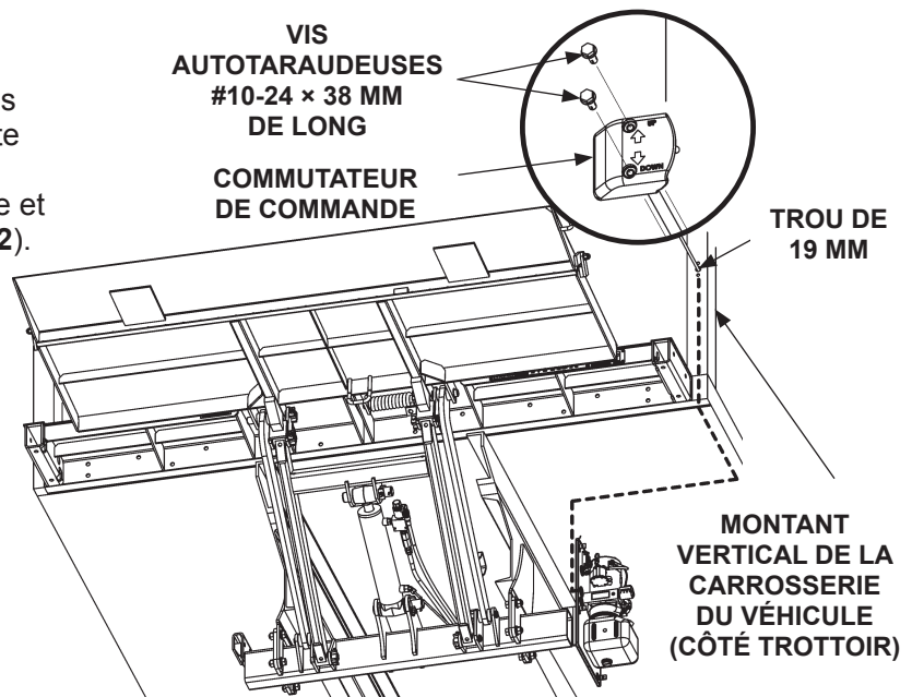
CÂBLAGE DU COMMUTATEUR DE COMMANDE FIG. 45-2
