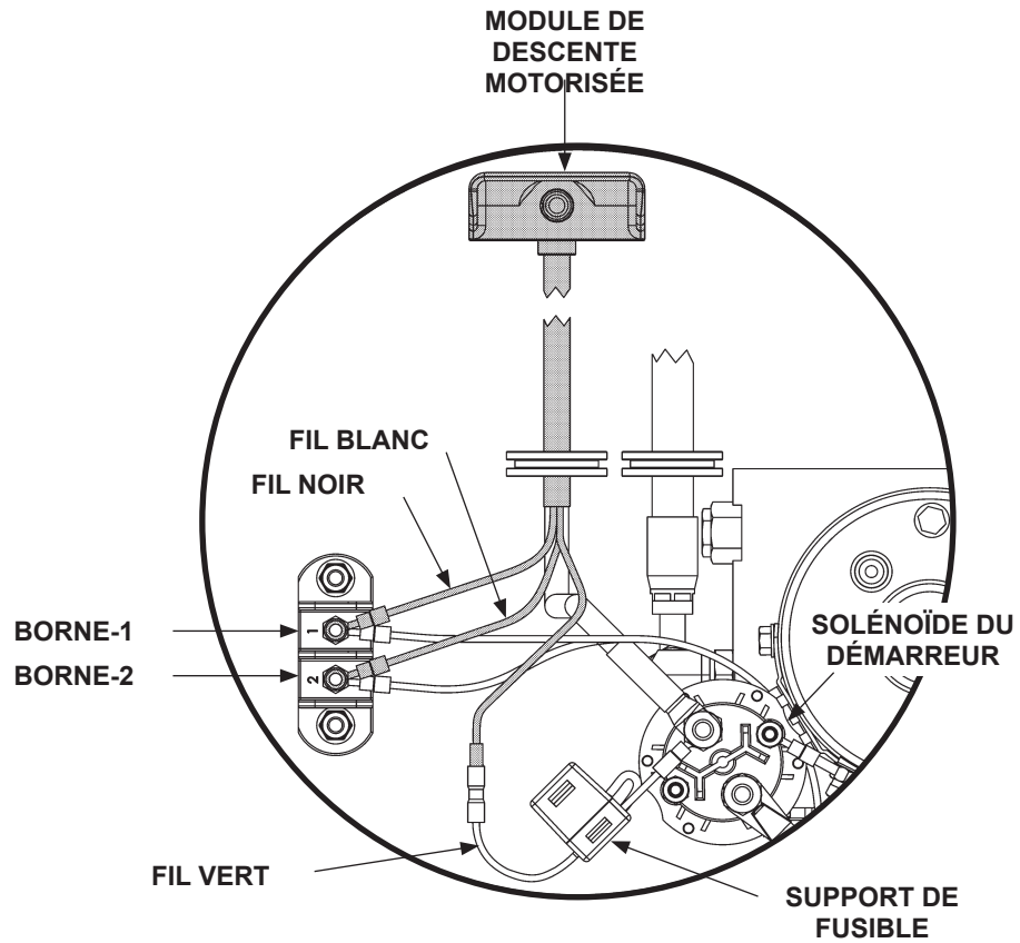
COMMUNTEUR DE COMMANDE CONNECTÉ À L'ASSEMBLAGE DE LA POMPE À DESCENTE MOTORISÉE FIG. 47-1
