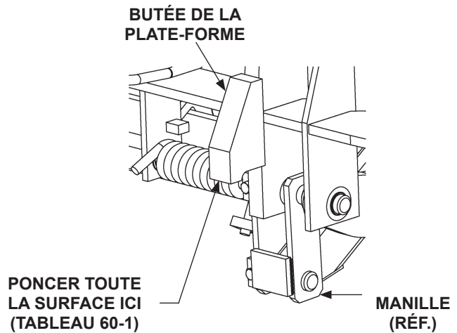
LA POINTE DE L'ÉLÉMENT RABATTABLE NE TOUCHE PAS LE SOL FIG. 60-2
