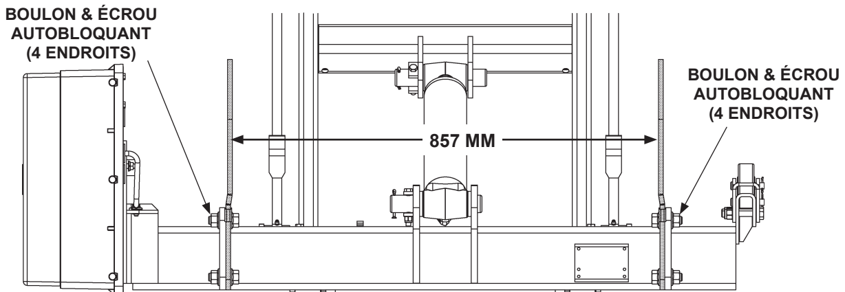
PLAQUES DE MONTAGE BOULONNÉES À 857 MM (GALVANISÉES) FIG. 24-2
