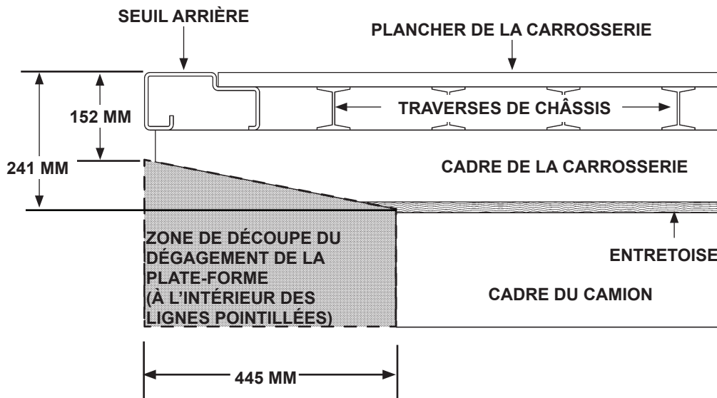
CADRE DU VÉHICULE DÉCOUPÉ (HAUTEURS DE PLANCHER DE 914 MM À 1117 MM) FIG. 13-2
