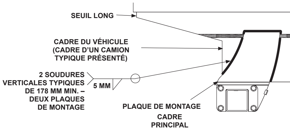
TE-25 & TE-30 PLAQUE DE MONTAGE SOUDÉE AU CHÂSSIS DU CAMION & BOULONNÉE AU CHÂSSIS PRINCIPAL FIG. 62-2
