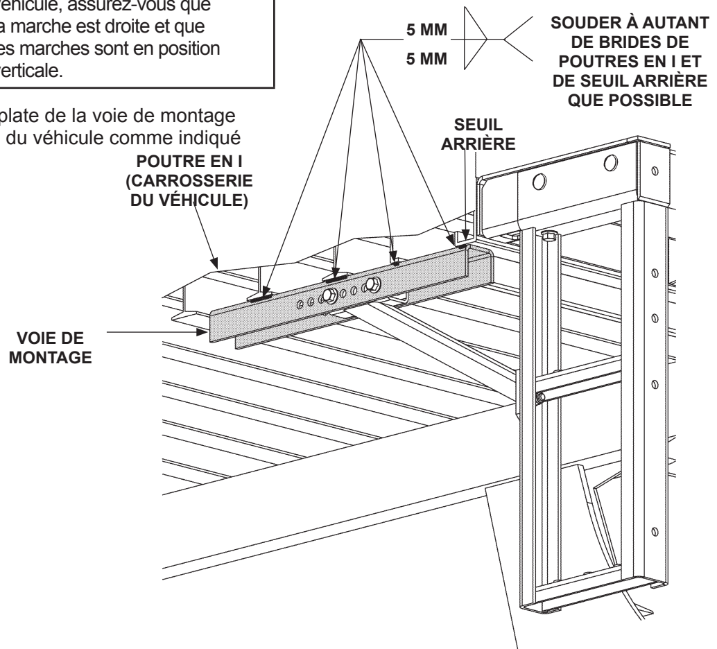
SOUDAGE PLAT DE LA VOIE DE MONTAGE À LA CARROSSERIE DU VÉHICULE (MARCHE DOUBLE GAUCHE INDICUÉE)
