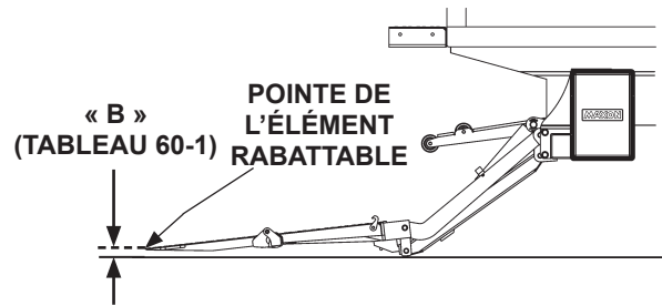
LA PLATE-FORME & LES MANILLES TOUCHENT LE SOL FIG. 60-1
