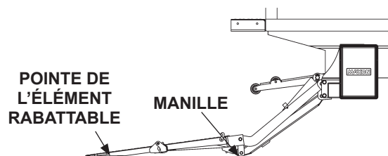
PONÇAGE DES BUTÉES DE LA PLATE-FORME (MANILLE DROITE INDICÉE) FIG. 60-3
