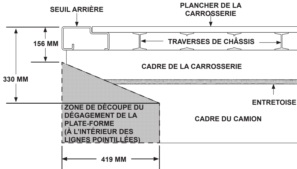
CADRE DU VÉHICULE DÉCOUPÉ (HAUTEURS DE PLANCHER DE 1067 MM À 1371 MM) FIG. 13-1
