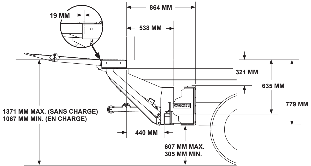
DÉGAGEMENTS POUR UNE INSTALLATION TE-20 À PLANCHER HAUT (PEINTE) FIG. 12-1
