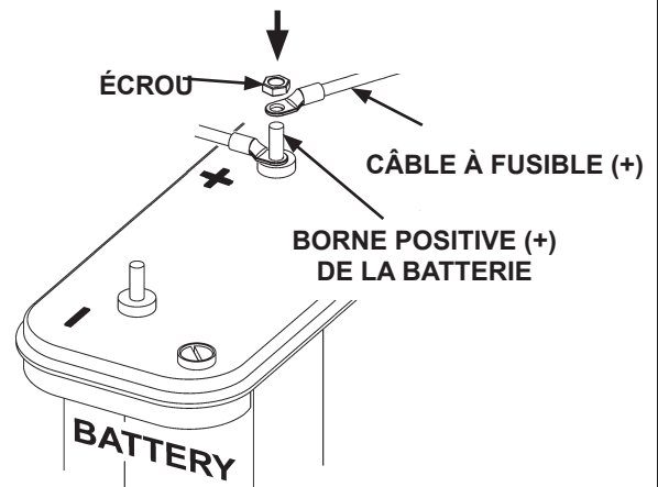
CONNEXION DU CÂBLE À FUSIBLE (+) FIG. 50-2
