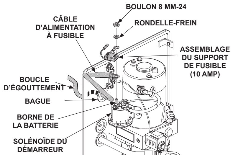
CONNEXION TYPIQUE DE CÂBLE D'ALIMENTATION À FUSIBLE (POMPE À DESCENTE PAR GRAVITÉ INDIQUÉE) FIG. 42-3
