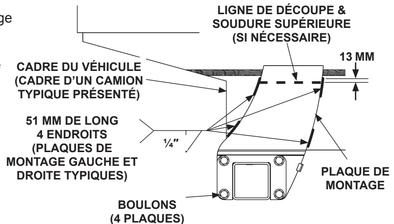
TE-25 & TE-30 SOUDER AU CADRE DU VÉHICULE (CÔTÉ DROIT MONTRÉ) FIG. 30-2
