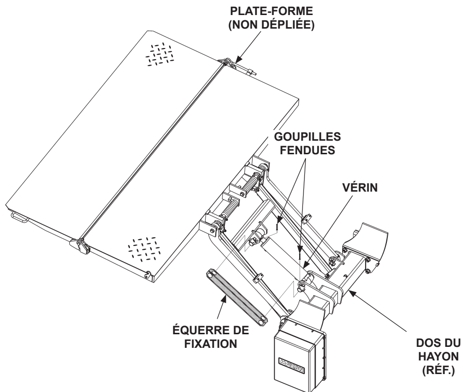
RETRAIT DE L'ÉQUERRE DE FIXATION FIG. 51-1
