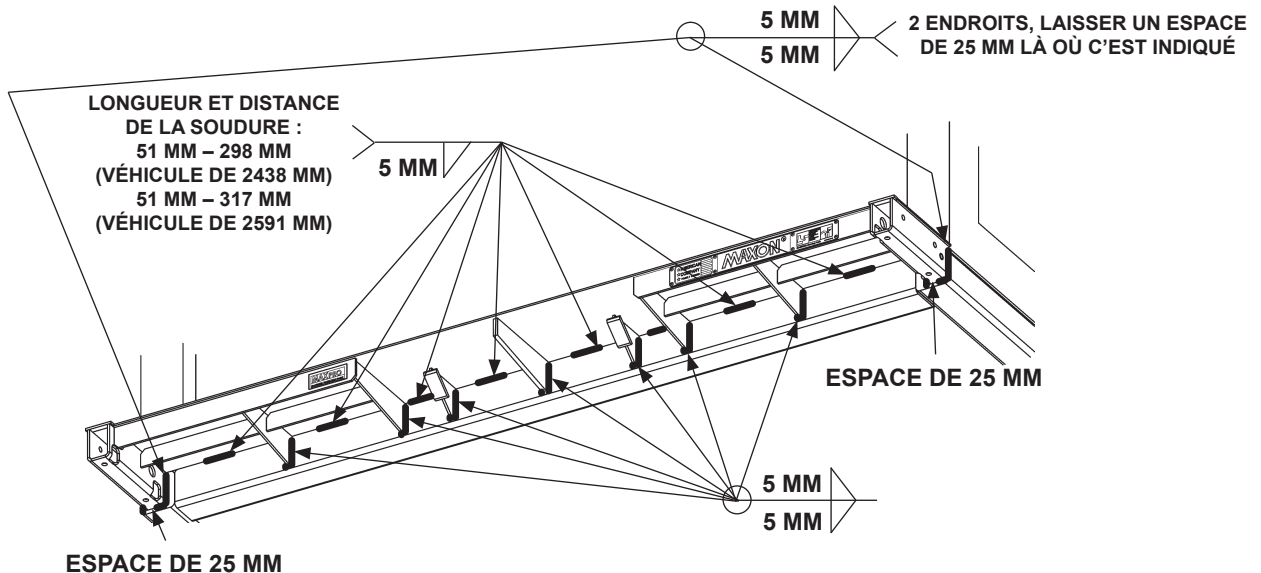
SOUDURES DE LA PLAQUE DE RALLONGE – VUES DE DESSOUS FIG. 18-2
