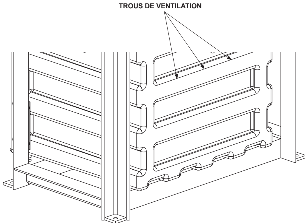
ASSEMBLAGE DU BOÎTIER DE LA BATTERIE (VUE ARRIÈRE MONTRÉE) FIG. 37-1
