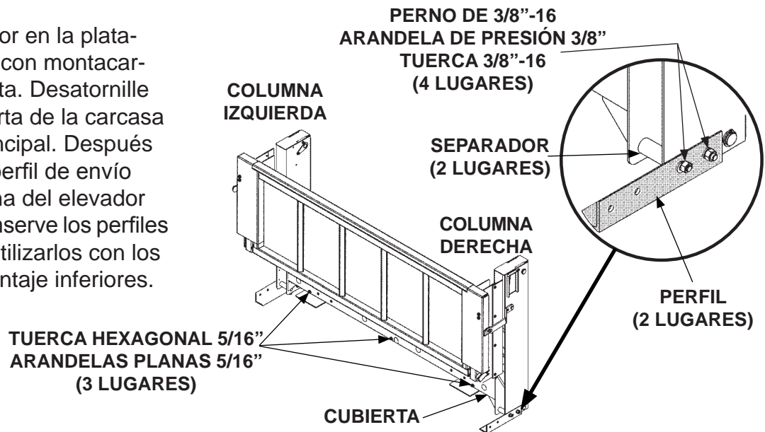
RETIRAR LOS PERFILES DE ENVÍO FIG. 35-1
