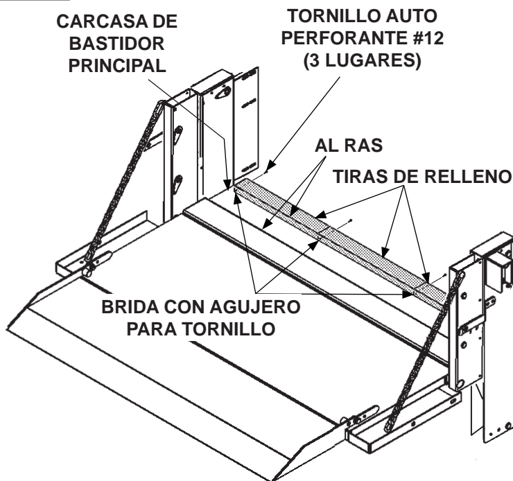
COLOCAR LAS TIRAS DE RELLENO FIG. 39-1
