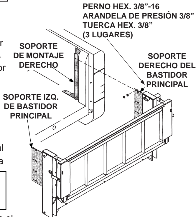
ATORNILLAR EL ELEVADOR AL SOPORTE DE MONTAJE DERECHO FIG. 40-2
