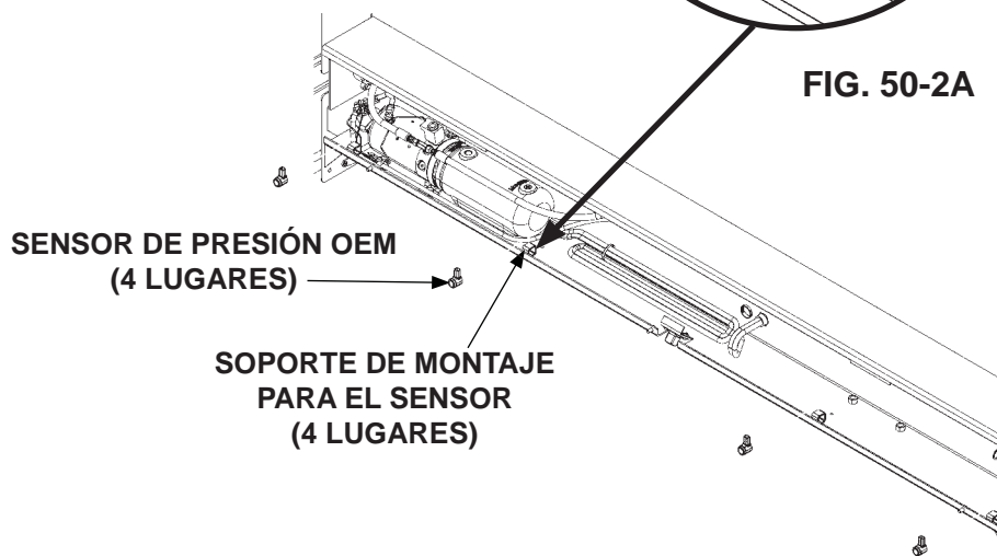
INSTALAR SENSORES (SI SE EQUIPA) FIG. 50-2
