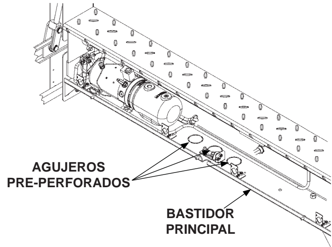
RETIRAR LOS AGUJEROS PRE-PERFORADOS EN LA CARCASA DEL BASTIDOR PRINCIPAL FIG. 36-1
