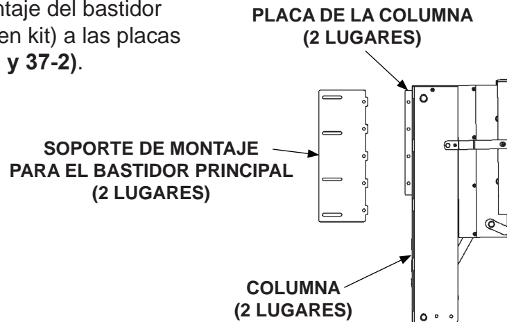
SE MUESTRA ELEVADOR C2 CON SOPORTES ATORNILLABLES PARA BASTIDOR PRINCIPAL FIG. 37-1
