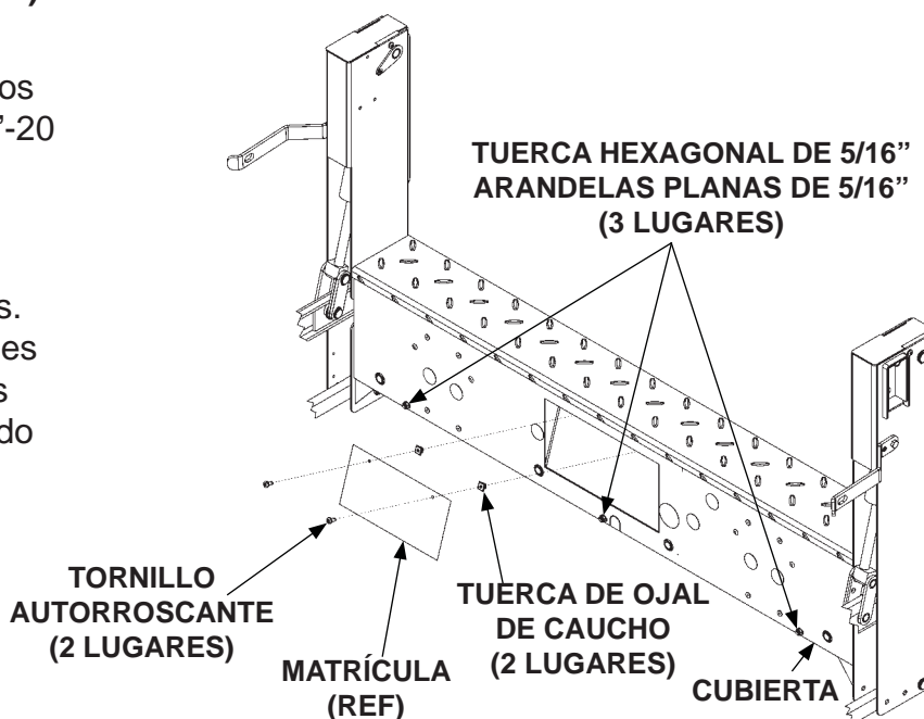
INSTALAR CUBIERTA Y MATRÍCULA (SE MUESTRA ELEVADOR C2) FIG. 53-2
