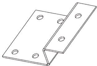
SOPORTE DE DISYUNTOR, GALVANIZADO N/P 295998-02 CANT. 1
