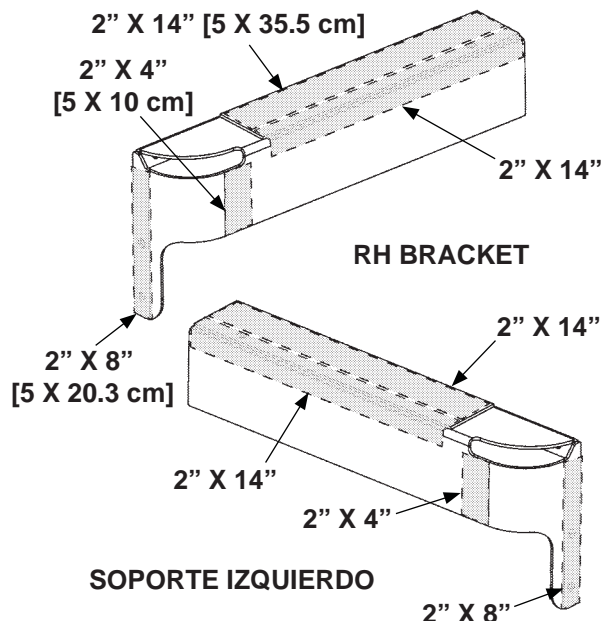
COLOCAR LA CINTA EN LOS SOPORTES DE MONTAJE FIG. 40-1
