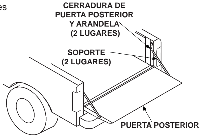
RETIRAR PUERTA POSTERIOR Y SOPORTES FIG. 38-1
