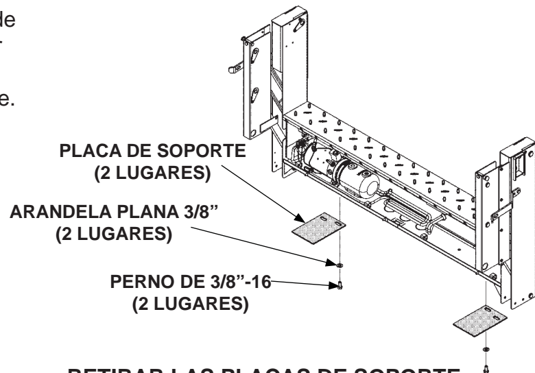
RETIRAR LAS PLACAS DE SOPORTE (LA PLATAFORMA NO SE MUESTRA) FIG. 35-2
