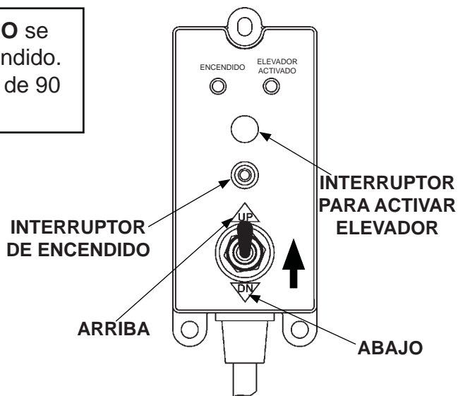
VERIFICAR OPERACIÓN DEL INTERRUPTOR Y ELEVAR LA PLATAFORMA FIG. 55-1
