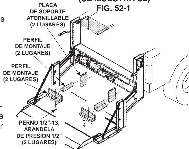
FABRICAR LOS SOPORTES INFERIORES PARA APOYAR AL ELEVADOR (SE MUESTRA C2) FIG. 52-2
