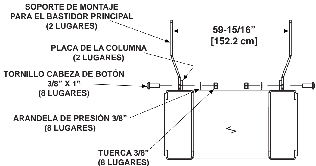
ATORNILLAR LOS SOPORTES DE MONTAJE PARA BASTIDOR PRINCIPAL A LAS COLUMNAS DEL ELEVADOR C2 (VISTA SUPERIOR) FIG. 37-2
