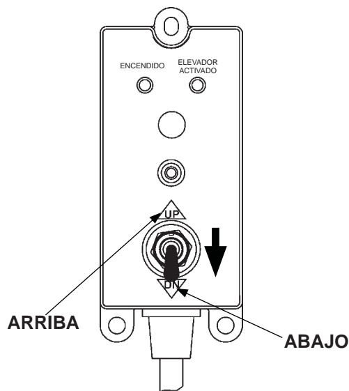
UTILIZAR INTERRUPTOR PARA DESCENDER LA PLATAFORMA FIG. 55-2
