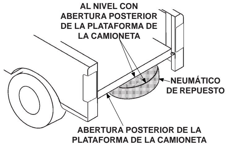
NEUMÁTICO DE REPUESTO Y TUBO DE ACCESO EN LA PLATAFORMA POSTERIOR DE LA CAMIONETA FIG. 36-1
