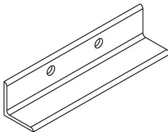
PERFIL DE ENVÍO N/P 289543-02 CANT. 2
