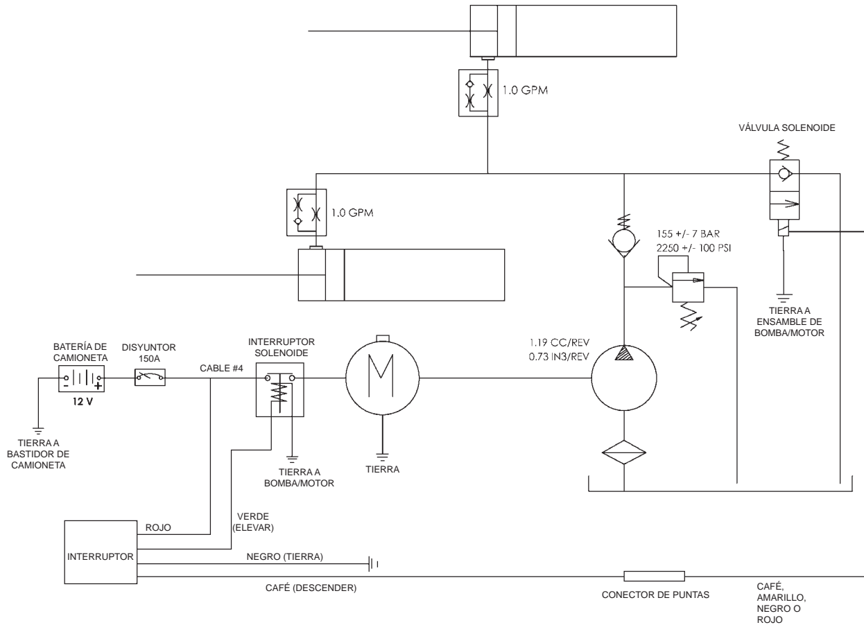
DIAGRAMA DE SISTEMAS ELÉCTRICOS E HIDRÁULICOS PARA ELEVADOR C2 FIG. 43-1
