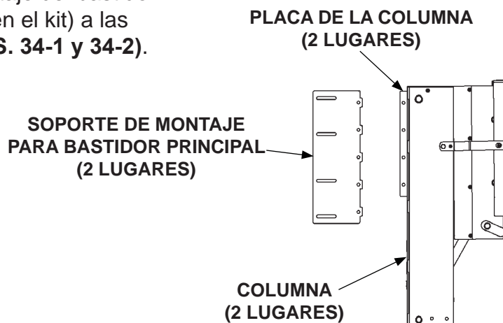
SE MUESTRA ELEVADOR C2 CON SOPORTES DE MONTAJE PARA ATORNILLARSE EN EL BASTIDOR PRINCIPAL FIG. 34-1
