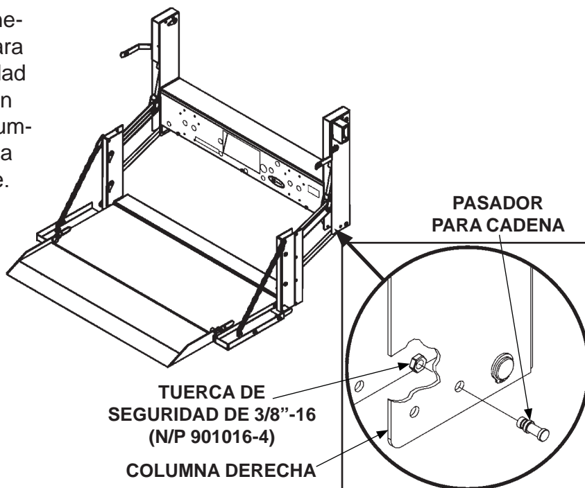
INSTALAR PASADOR PARA CADENA EN LA COLUMNA DERECHA (SE MUESTRA ELEVADOR C2) FIG. 50-1
