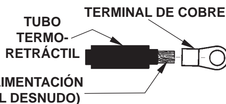
COLOCAR TERMINAL DE COBRE Y TUBO TERMORETRÁCTIL EN CABLE DE ALIMENTACIÓN FIG. 42-2
