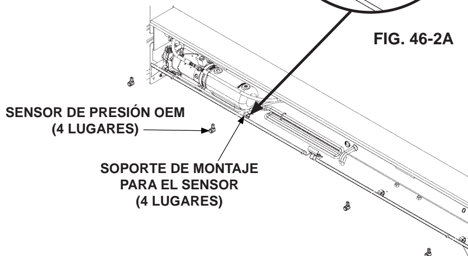
INSTALAR SENSORES (SI SE EQUIPA) FIG. 46-2
