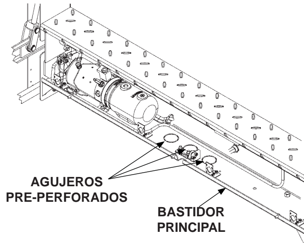
ABRIR LOS AGUJEROS PRE-PERFORADOS DE LA CARCASA DEL BASTIDOR PRINCIPAL FIG. 33-1
