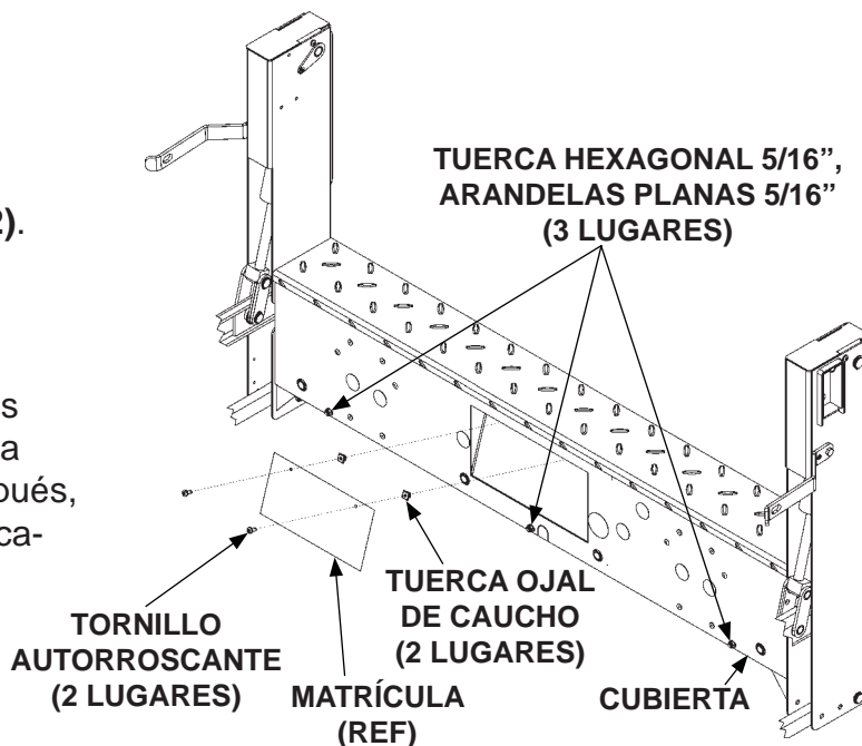
INSTALAR CUBIERTA Y MATRÍCULA (SE MUESTRA ELEVADOR C2) FIG. 49-2
