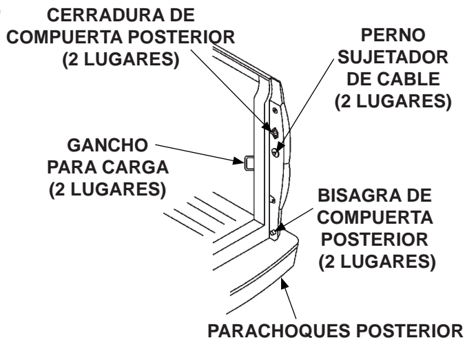
RETIRAR COMPUERTA POSTERIOR Y SOPORTES FIG. 35-1
