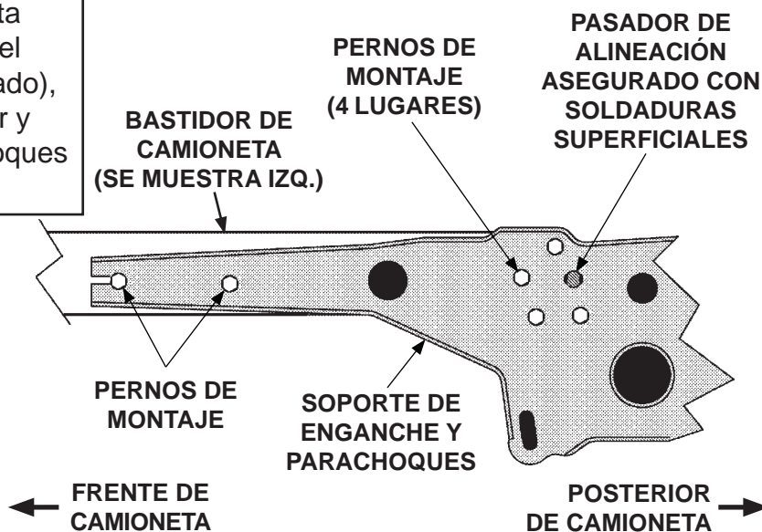
ENGANCHE Y SOPORTE POSTERIOR DE PARACHOQUES VISTO DESDE EL LADO IZQUIERDO EXTERIOR DEL BASTIDOR DE LA CAMIONETA FIG. 35-2
