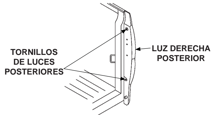
TORNILLOS DE MONTAJE DE LUCES POSTERIORES (SE MUESTRA LUZ DERECHA POSTERIOR) FIG. 37-1
