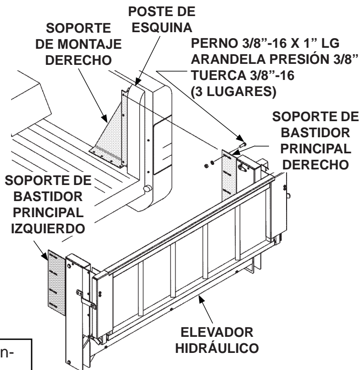
ATORNILLAR EL ELEVADOR AL SOPORTE DE MONTAJE DERECHO FIG. 38-1
