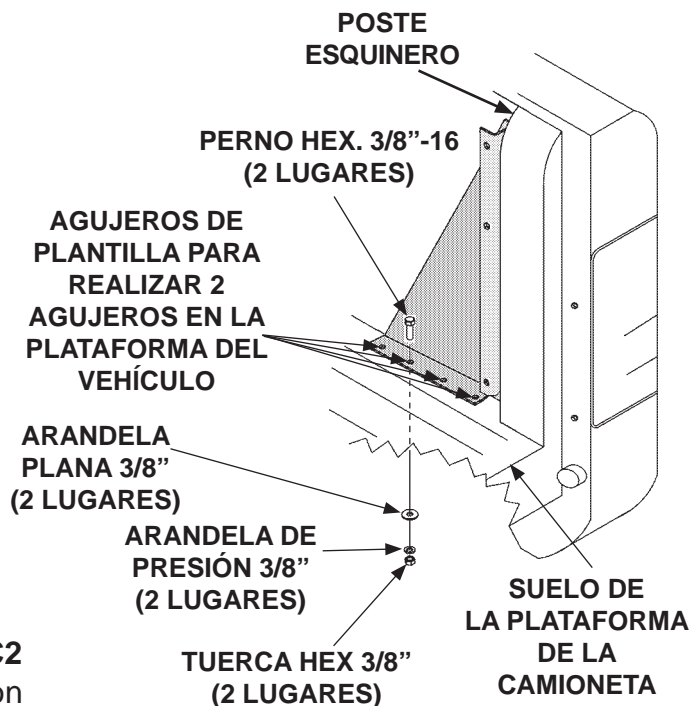
ATORNILLAR SOPORTE DE MONTAJE DERECHO A LA PLATAFORMA DE LA CAMIONETA (NO SE MUESTRA ELEVADOR) FIG. 39-1
