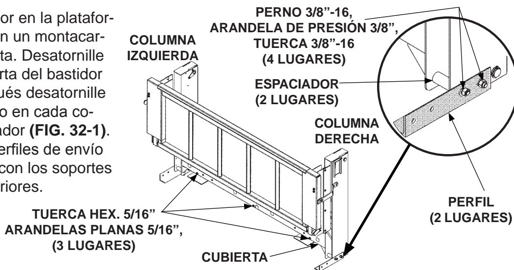
RETIRAR PERFILES DE ENVÍO FIG. 32-1
