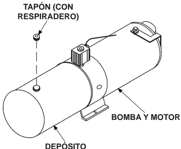
INSTALAR EL TAPÓN DE VENTILACIÓN EN EL DEPÓSITO DE LA BOMBA FIG. 49-1
