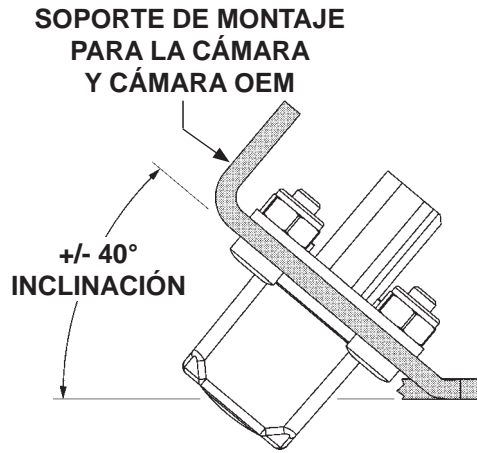
AJUSTAR EL ÁNGULO DE LA CÁMARA FIG. 46-1
