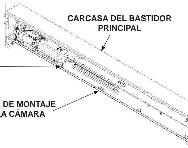
UBICACIÓN DEL SOPORTE DE LA CÁMARA Y DEL SENSOR FIG. 44-1
