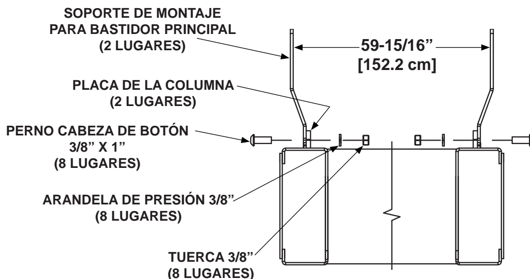
ATORNILLAR SOPORTES DE MONTAJE PARA BASTIDOR PRINCIPAL A LAS COLUMNAS EN ELEVADOR C2 (VISTA SUPERIOR) FIG. 34-2
