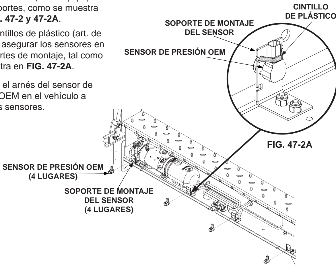
INSTALAR SENSORES (SI SE EQUIPA) FIG. 47-2
