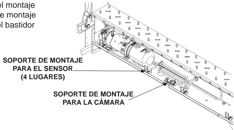
UBICACIÓN DEL SOPORTE DE LA CÁMARA Y DEL SENSOR FIG. 46-1
