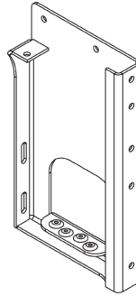
Escalón, der. sencillo, atornillable N/P 285898-04 (pintado) N/P 285898-04G (galv.) cant. 1
