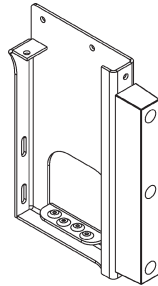
Escalón, der. sencillo, atornillable N/P 285898-04 (pintado) N/P 285898-04G (galv.) cant. 1
