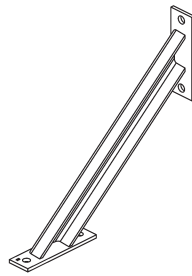
Soporte derecho N/P 285899-02 (pintado) N/P 285899-02G (galv.) cant. 1
