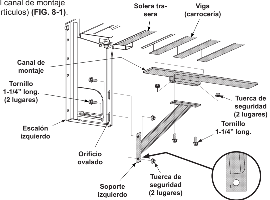
Atornillar soportes a canal de montaje y escalera (se muestra escalera y soporte de lado izquierdo) FIG. 8-1
