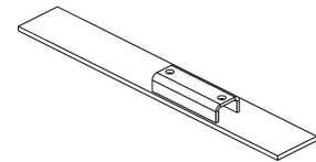
Canal de montaje, der. N/P 285897-02 (pintado) N/P 285897-02G (galv.) cant. 1
