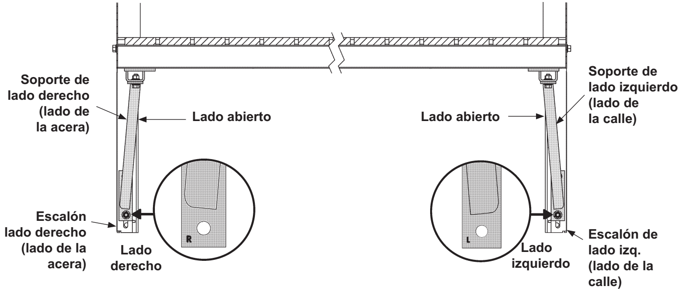
Instalación correcta de escaleras y soportes (se muestra vista trasera)
